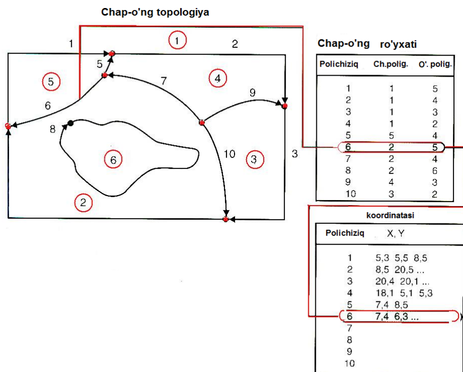
4.23-rasm. Poligonlarni chegaralash chiziqlari topologiyasi (Manba: Longley, 2005)
