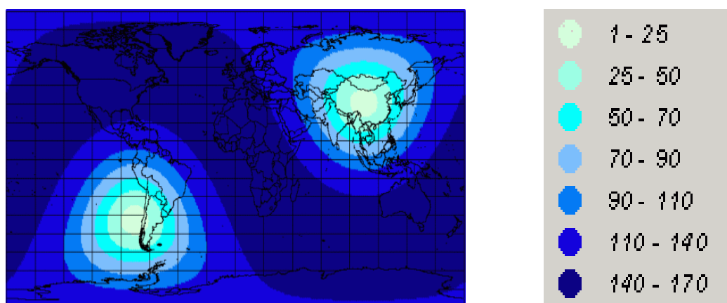
2.6-rasm. Dunyo hududlari bo'yicha SK42 va WGS84 sistemalarining farqi (Manba: Internet)
