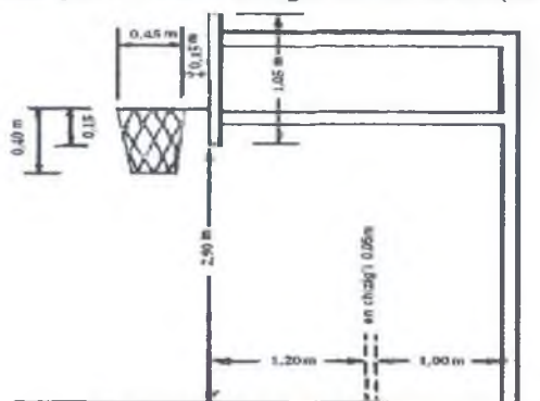
38-rasm. Halqa shchit qurilmasi.
