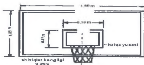
39-rasm. Shchit. Uning o'lchovlari.
