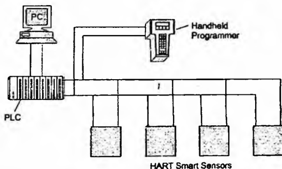
15.3-rasm. HART protokolidan ko'p nuqtali aloqalar.
