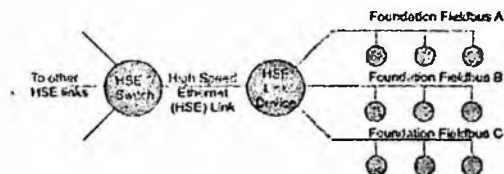
16.16-rasm. Yuqori tezlik Ethernet va Foundation Fieldbus.
