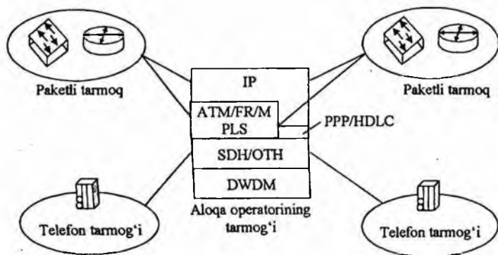
10.15-rasm. Aloqa operatori tarmog'ining ko'p bosqichli tarkibi.
