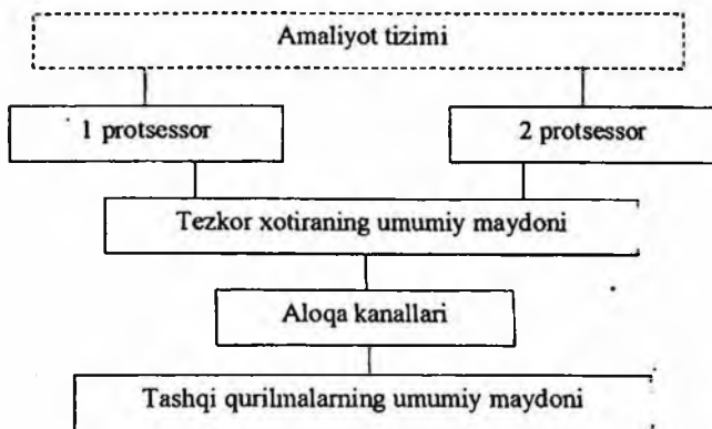
2.4-rasm. Hisoblash tizimidagi protsessorlarning muloqot sxemasi.
