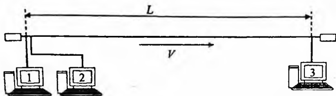
5.20-rasm. Paketni minimal uzunligini hisoblash.
