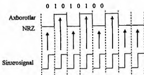
6.12-rasm. NRZ kodida sinxrosignal yordamida axborotlarni uzatish.
