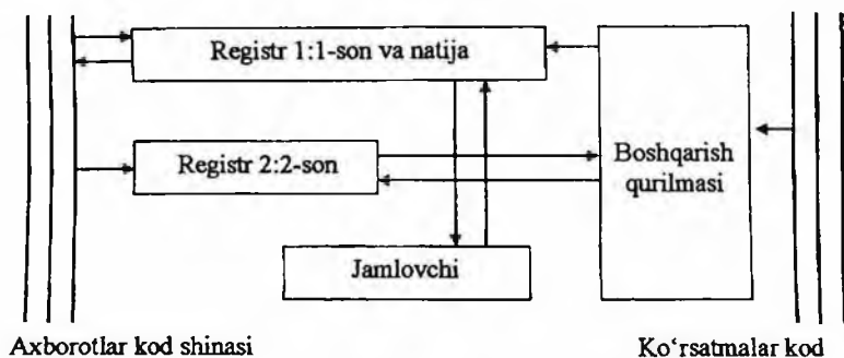
1.11-rasm. Arifmetik-mantiqiy qurilmaning funksional sxemasi.
