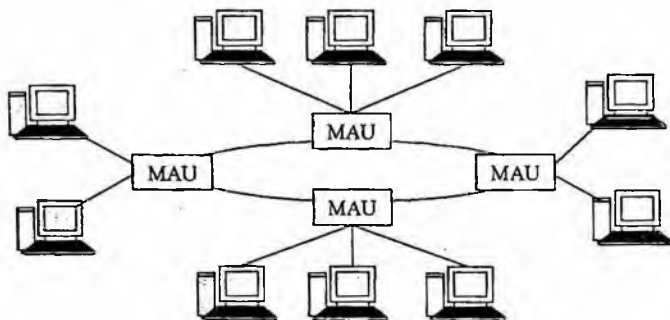
7.3-rasm. Token-Ring tarmog'ining yulduzsimon aylana topologiyasi.
