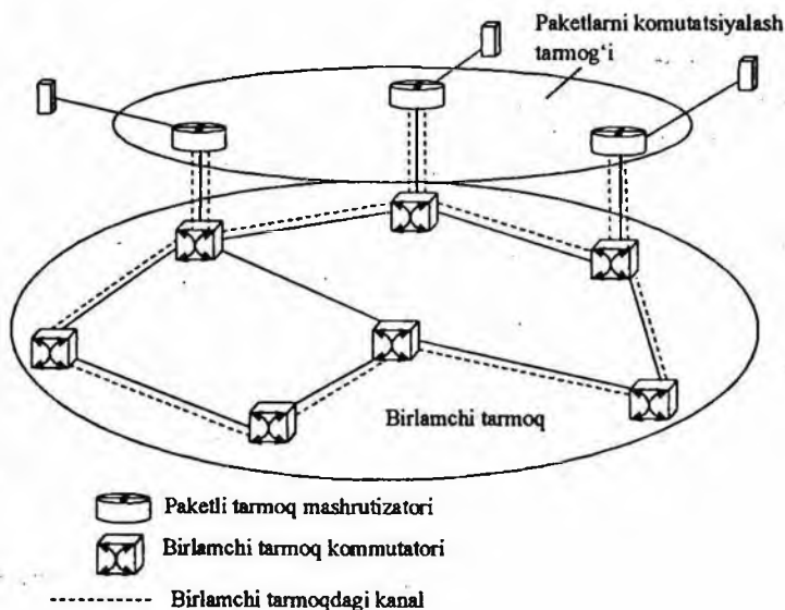
10.1-rasm. Birlamchi tarmoq orqali marshrutizatorlarni ulanishi.
