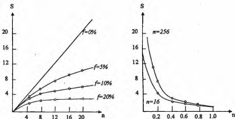
3.2-rasm. Tezlatishni bog'liqlik grafigi: a-ketma-ket hisoblashlar ulushi; b-protsessorlar soni.
