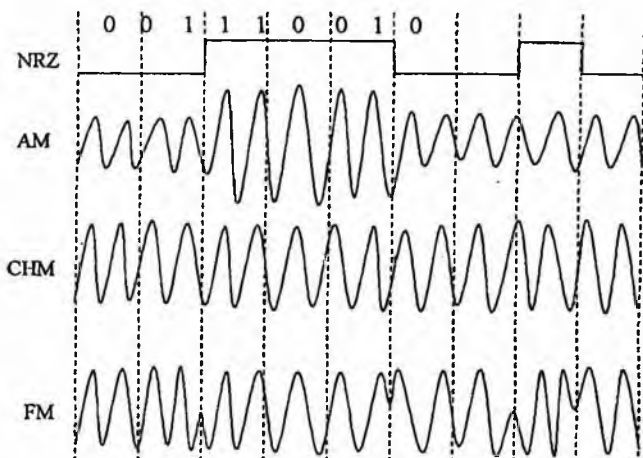
6.14-rasm. Raqamli axborotni analogli kodlash.
