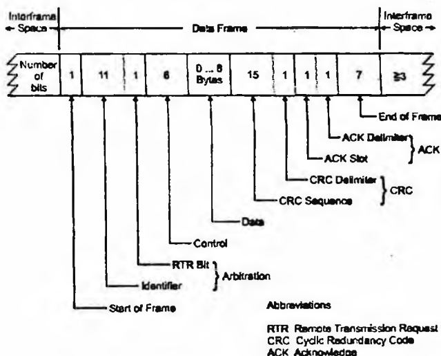
16.10-rasm. CANbus paketi.
