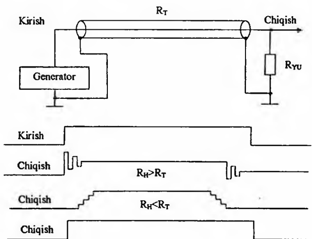
6.4-rasm. Elektr kabellari orqali signallarni uzatish.
