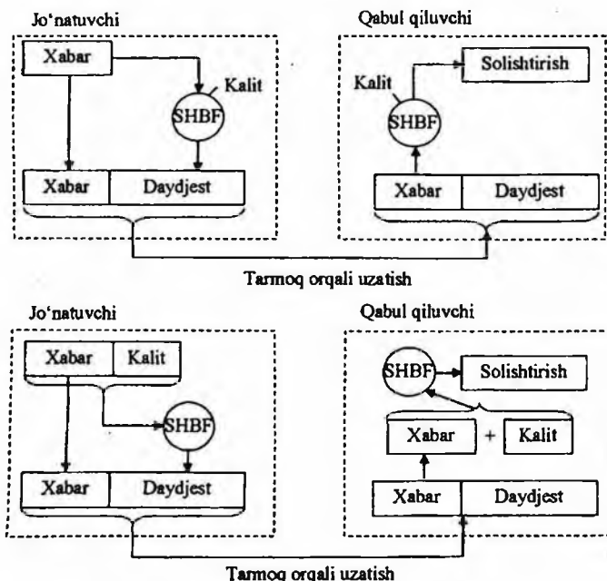
12.4-rasm. Shifrlashning bir tomonlama funksiyalari.
