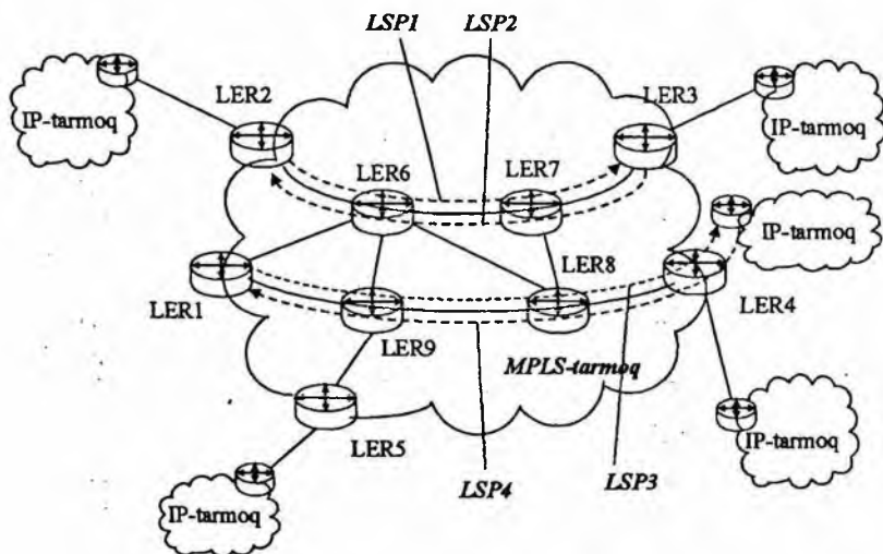
10.12-rasm. MPLS tarmog'i.
