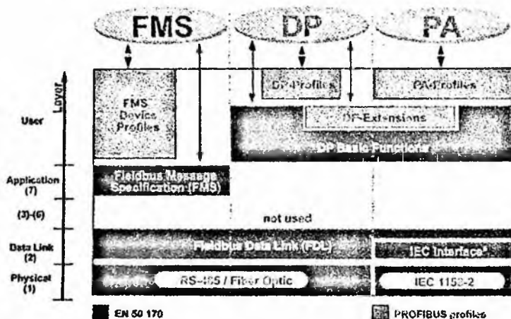
16.11-rasm. Profiliniya tuzilishi.
