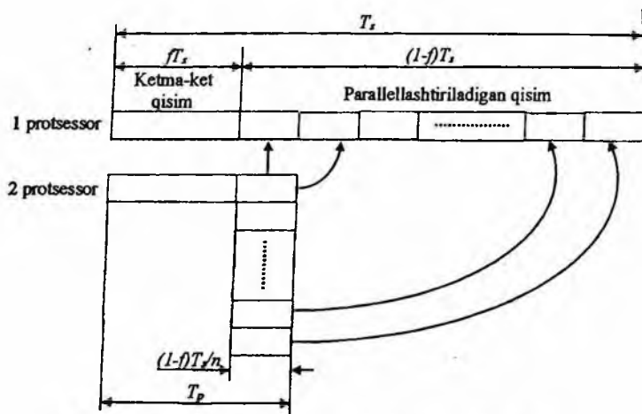
3.1-rasm. Amdal qonunida masalaning qo'yilishi.
