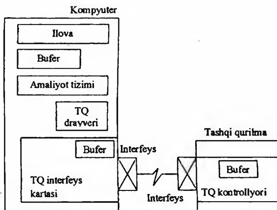
9.7-rasm. Kompyuterning tashqi qurilmalar bilan aloqasi.
