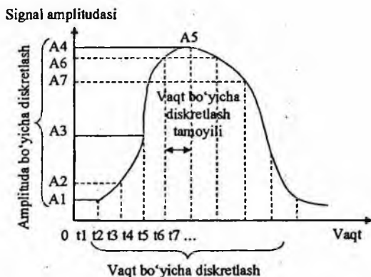
10.8-rasm. Uzluksiz jarayonni diskret modulatsiyalash.
