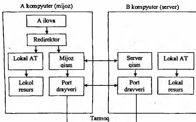
9.6-rasm. Ikki kompyuter dasturiy komponentlarining aloqasi.
