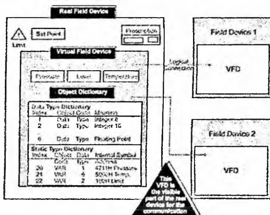
16.13-rasm. Virtual soha qurilmasi(VFD) obyekt lug'ati bilan.
