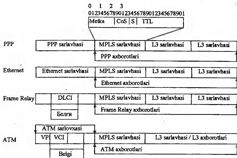
10.13-rasm. Bir necha MPLS texnologiya turlarining sarlavhalarini o'lashlari.
