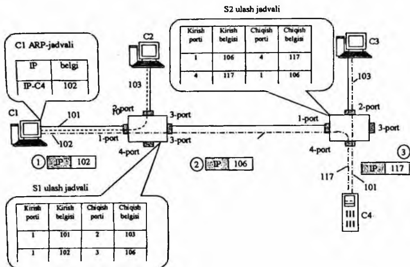
10.5-rasm. Virtual kanal bo'ylab kadrlarning harakatlanishi.
