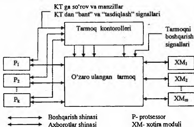
3.3-rasm. Markazdan boshqariladigan tarmoq tarkibi.
