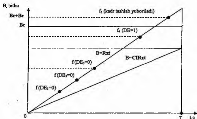
10.6-rasm. Foydalanuvchining xatti-harakatiga tarmoqning javobi.
