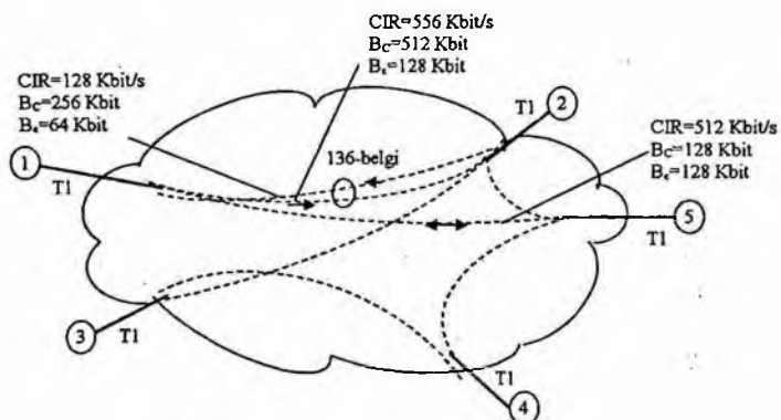
10.7-rasm. Frame Relay tarmog'idagi xizmat ko'rsatishga misol.
