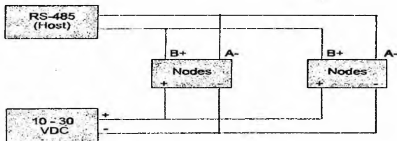
14.2-rasm. RS-485 ma'lumot uzatish kanali.
