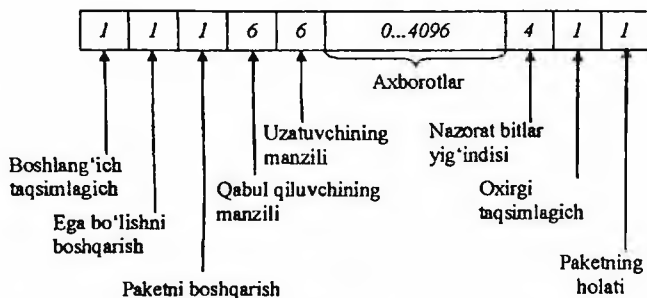
7.10-rasm. Token-Ring tarmoq paketining o'lchami (maydon uzunliklari baytda berilgan).
