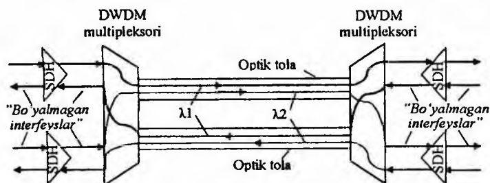
10.4-rasm. Bitta tolada turli uzunlikdagi to'liqlarni multiplesirlash tamoyili.
