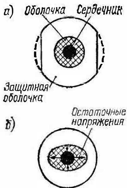
Рис. 113. Получение волокон с двойным лучепреломлением в сердечнике
