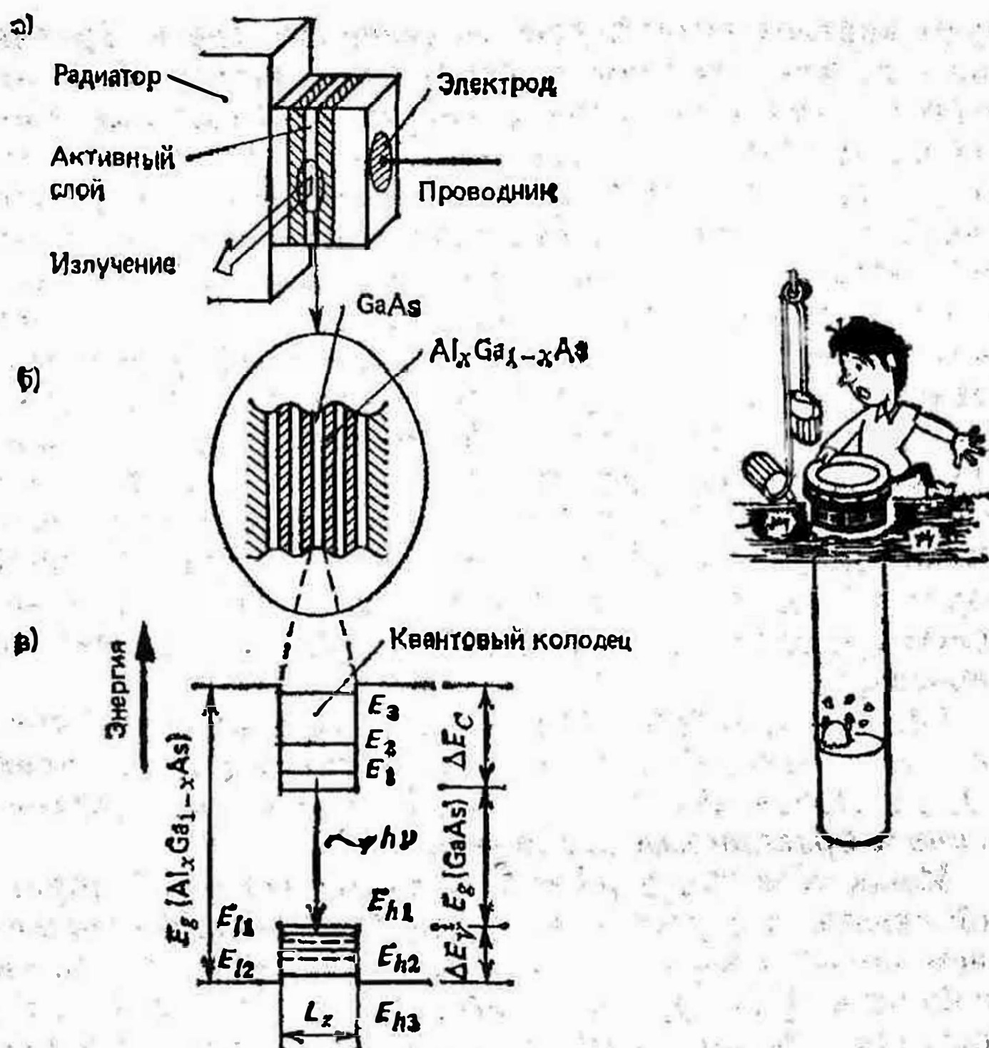
Рис. 56. Полупроводниковый лазер с мультиквантовым колодцем: а — двойная гетероструктура; б — активный слой (слой с мультиквантовым колодцем); в — дискретные уровни в квантовом колодце
