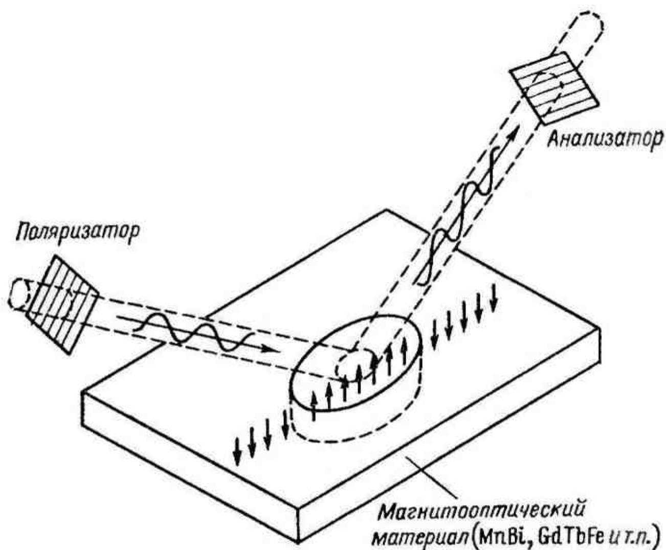
Рис. 19. Считывание оптической памяти с использованием эффекта Керра
