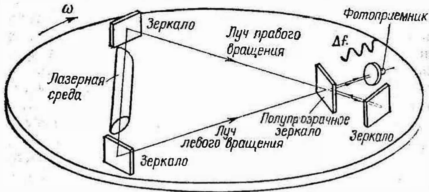
Рис. 138. Гироскоп на кольцевом лазере
