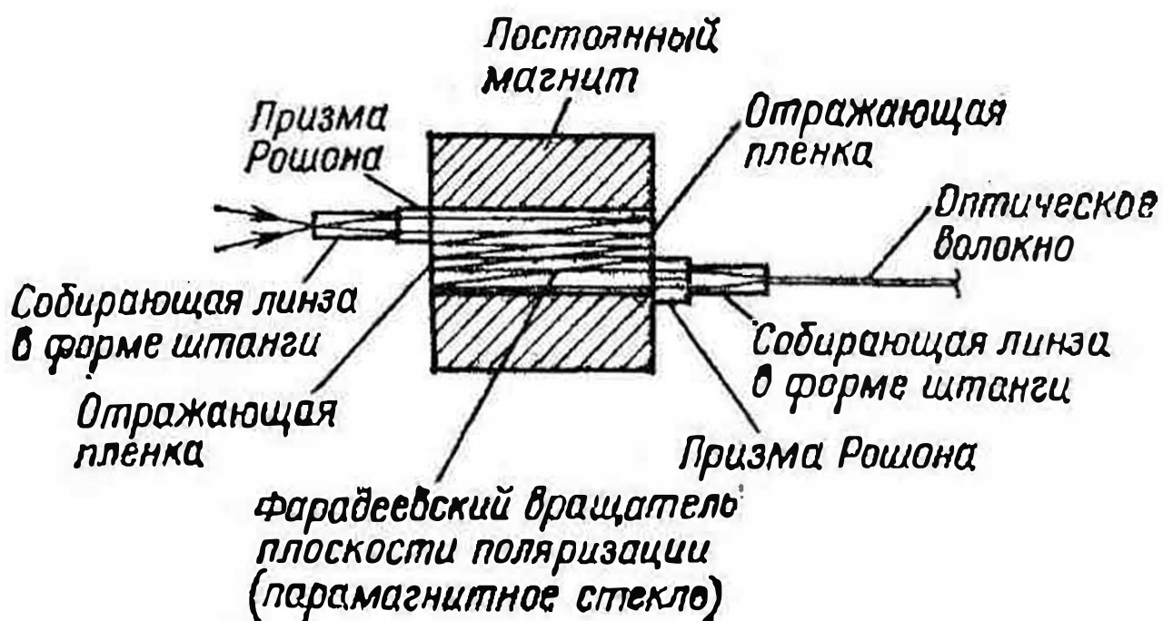
Рис. 107. Оптический вентиль для волн 0,8 мкм (OQE 78—133)
