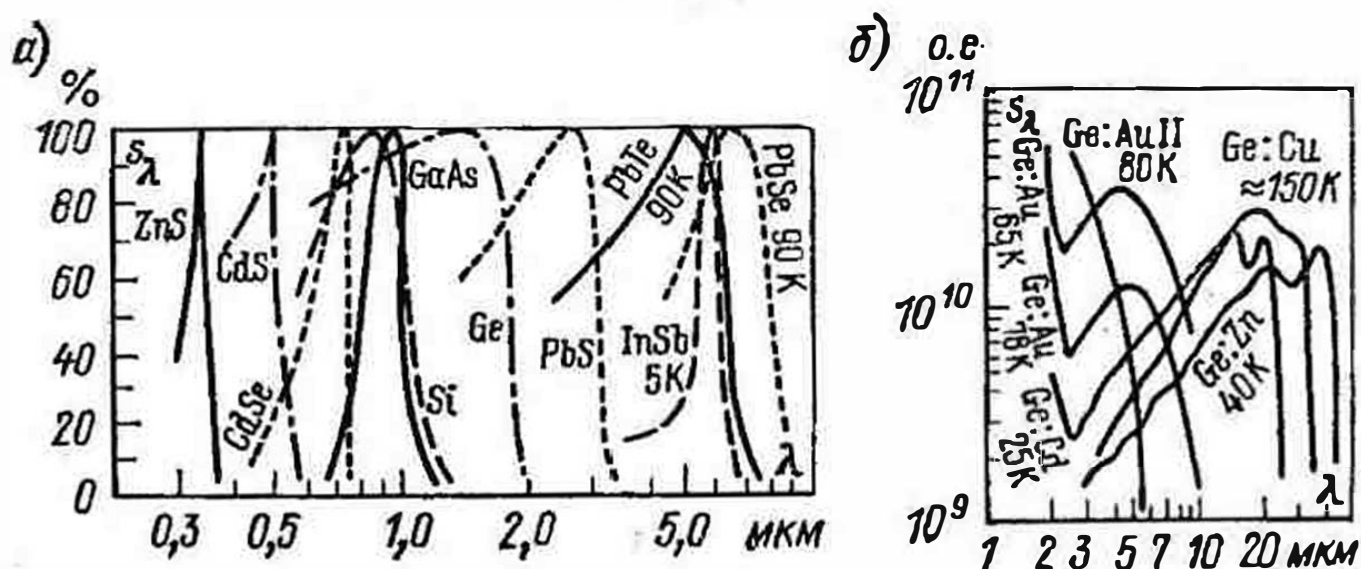
Рис. 29. Спектральная чувствительность фотопроводящих материалов
