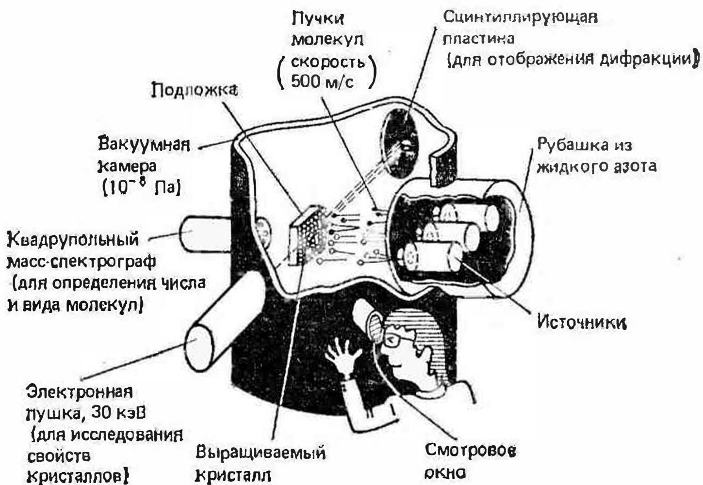
Рис. 43. Молекулярно-лучевая эпитаксия
