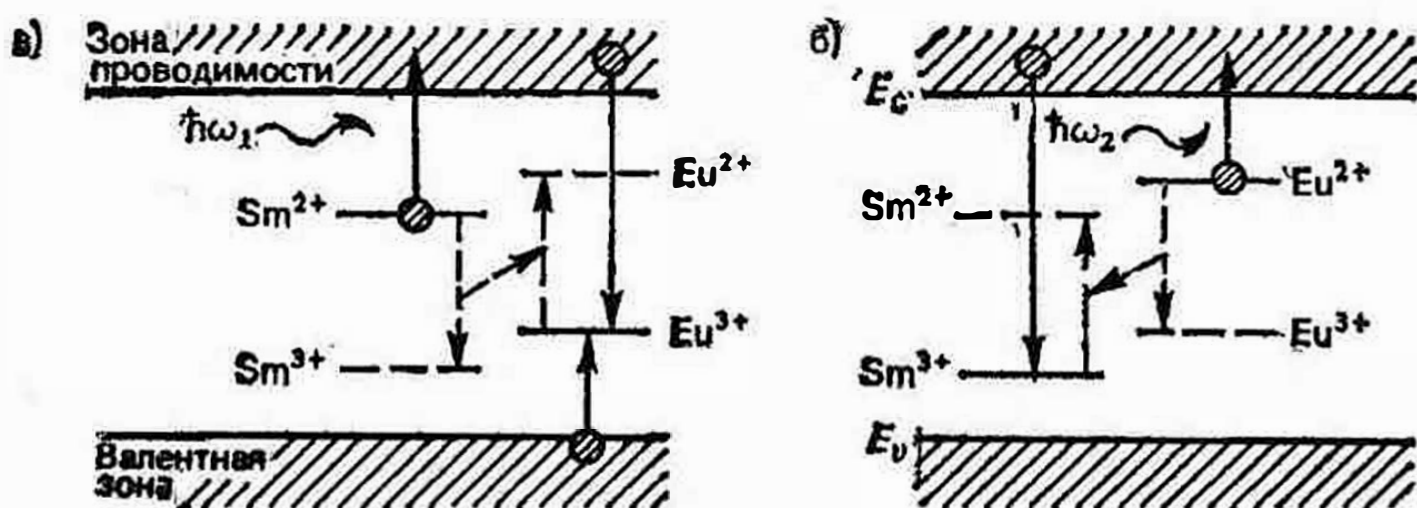
Рис. 24. Фотохромный эффект в кристалле \text{CaF}_2:\text{Sm}, \text{Eu} : а — облучение ультрафиолетом; б — облучение видимым светом
