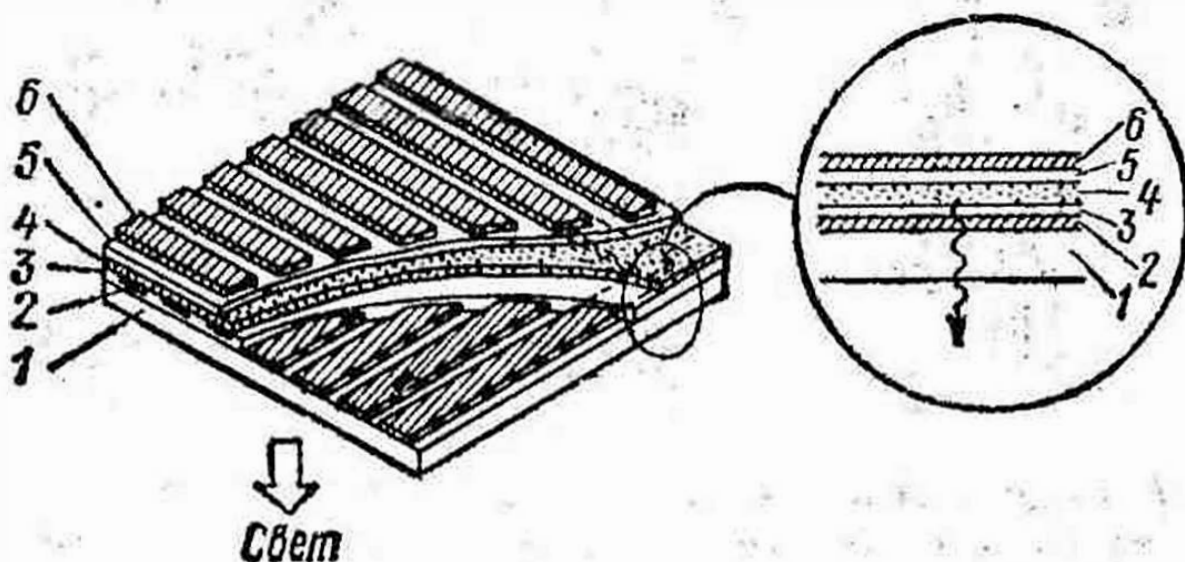
Рис. 76. Электролюминесцентный дисплей 1 — стеклянная пластина; 2 — прозрачный электрод; 3 — слой диэлектрика ( \text{Si}_3\text{N}_4 ); 4 — активный слой; 5 — слой диэлектрика ( \text{Y}_2\text{O}_3 ); 6 — электрод (Al)
