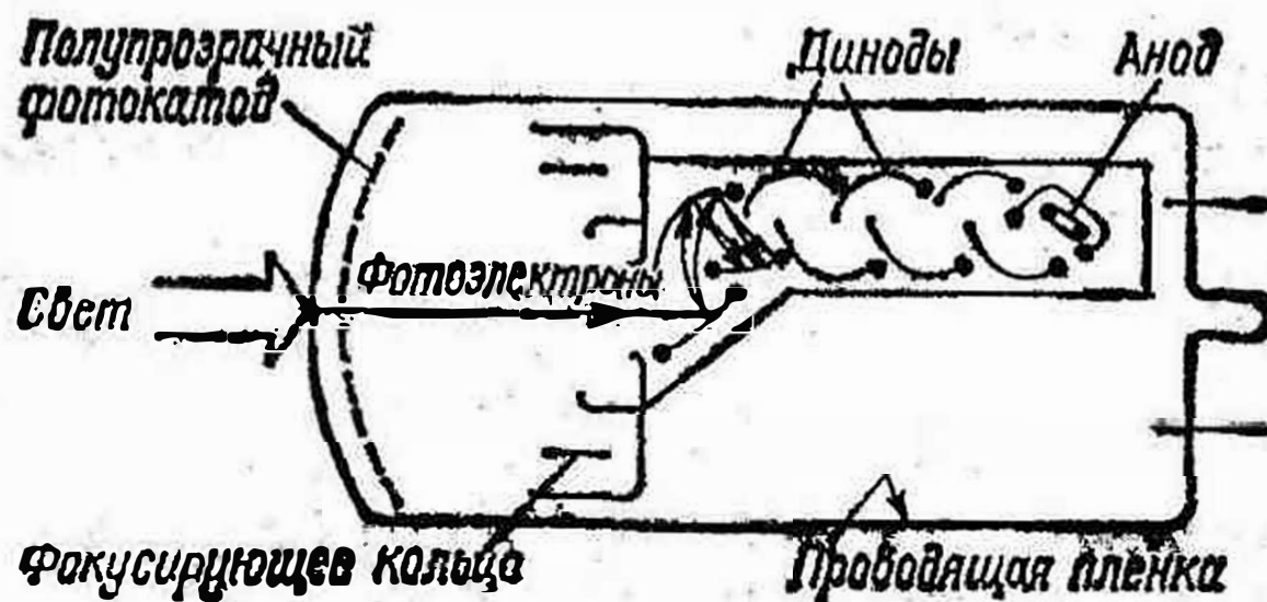
Рис. 82. Фотоумножитель
