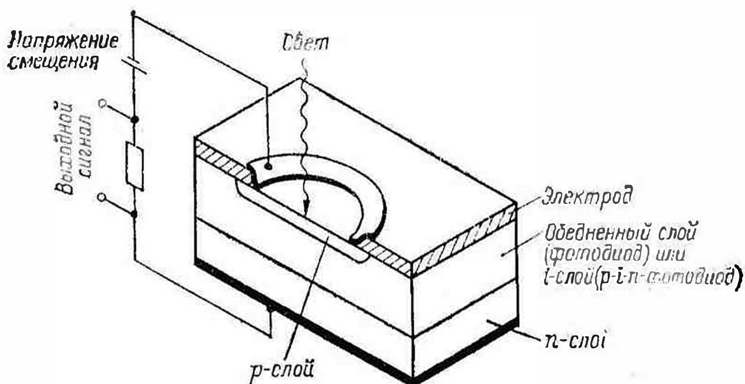
Рис. 84. Фотодиод и p-i-n -фотодиод
