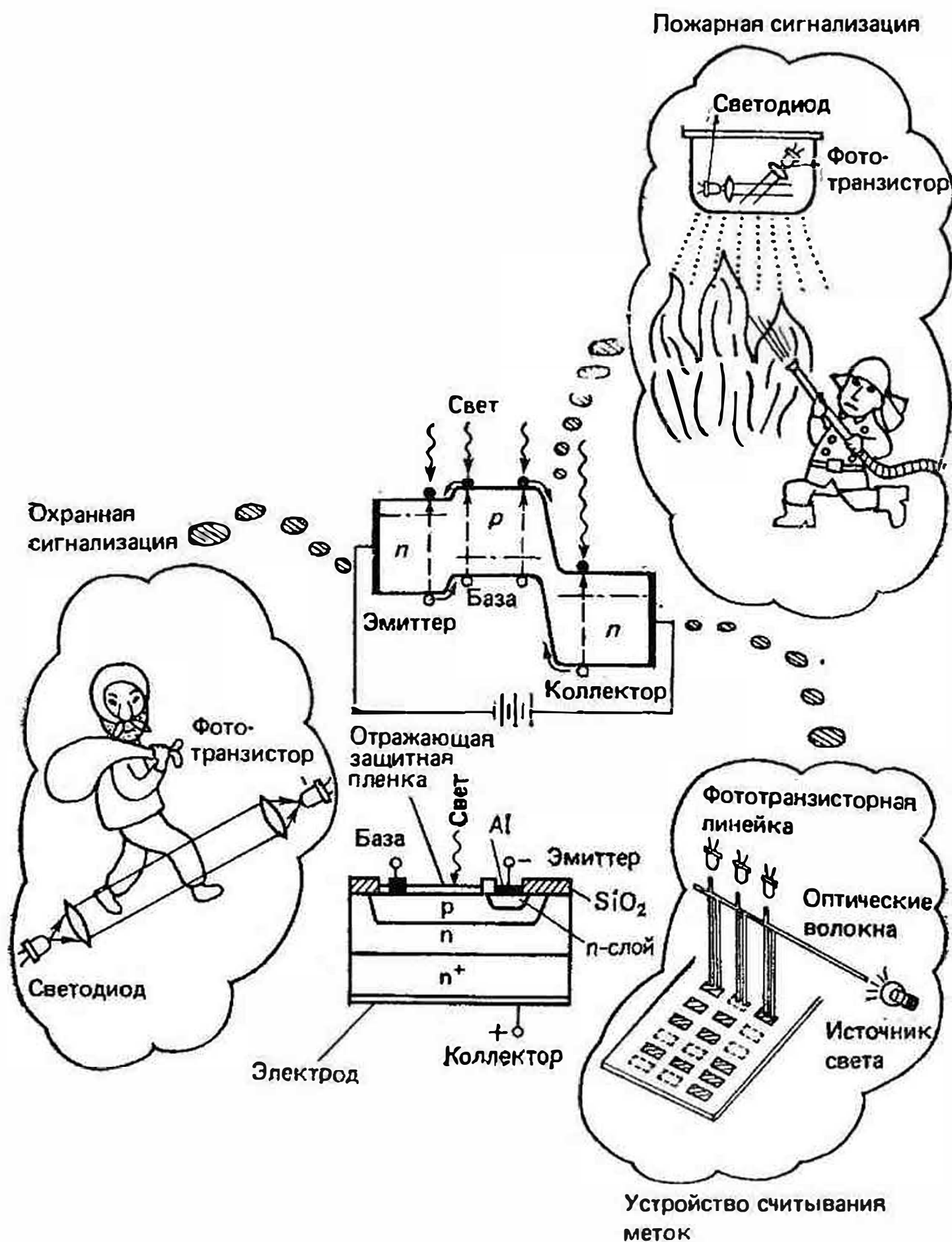
Рис. 87. Устройство и принцип работы фототранзистора
