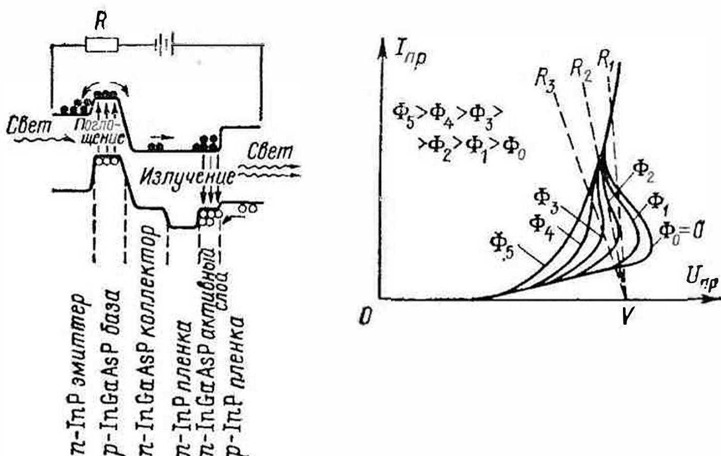
Рис. 89. Диаграмма энергетических уровней и вольт-амперная характеристика светодиода-фототиристора
