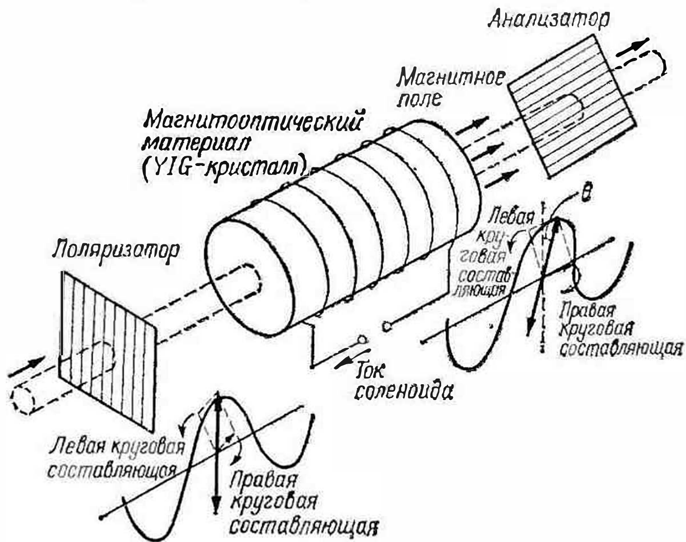
Рис. 18. Оптический модулятор на основе эффекта Фарадея
