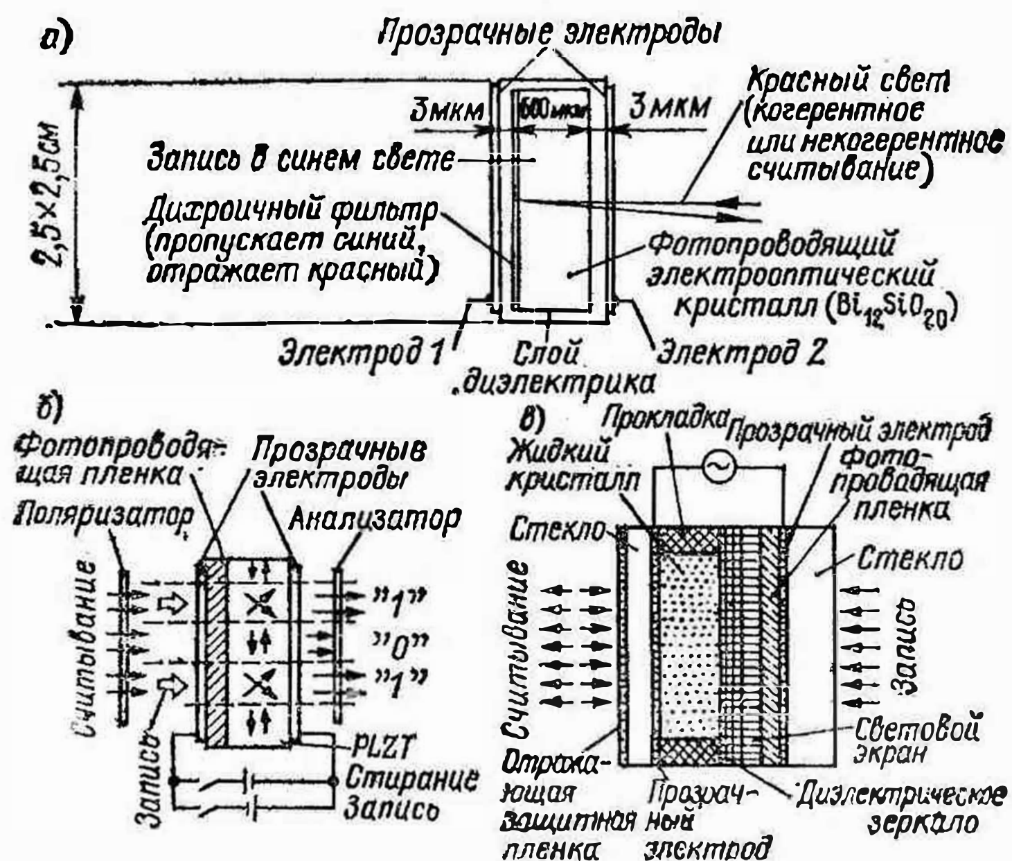
Рис. 99. Преобразователь некогерентного изображения в когерентное
