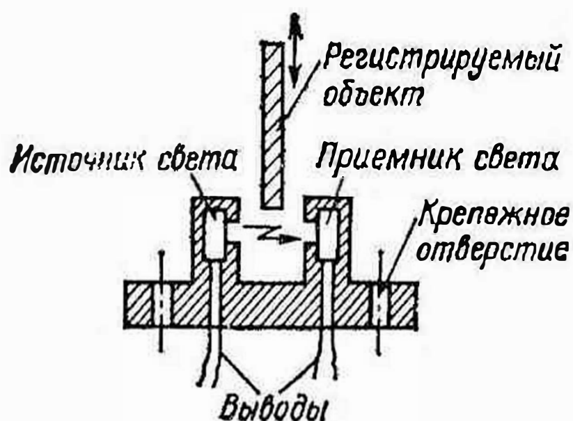
Рис. 105. Оптический прерыватель
