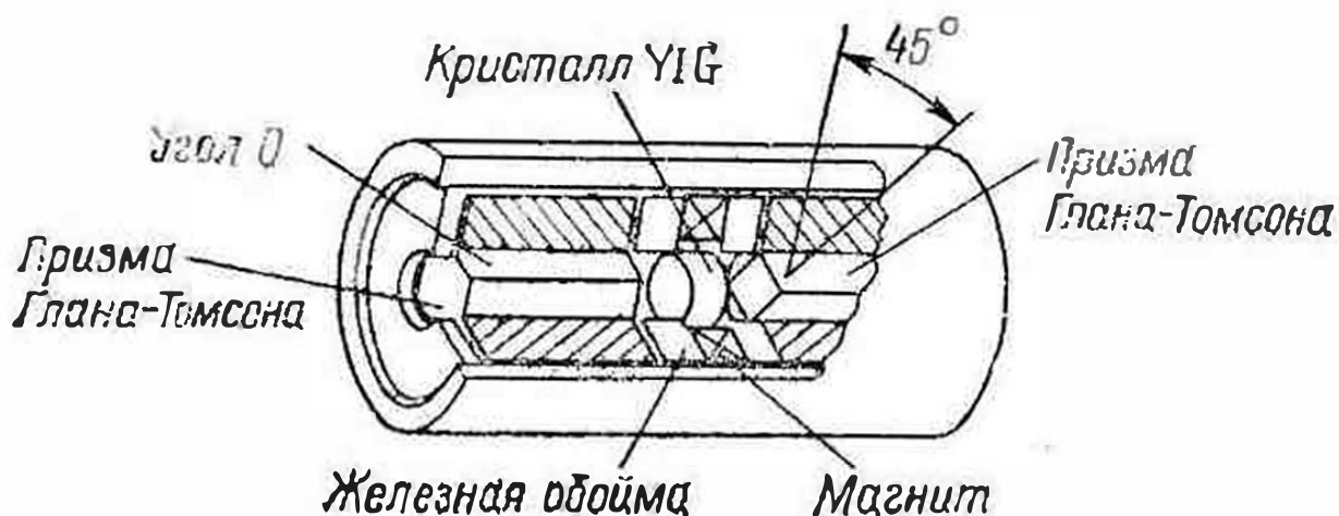
Рис. 108. Оптический вентиль (Iwamura a. oth., Ferrites Proc. ICF3 787, 1981)
