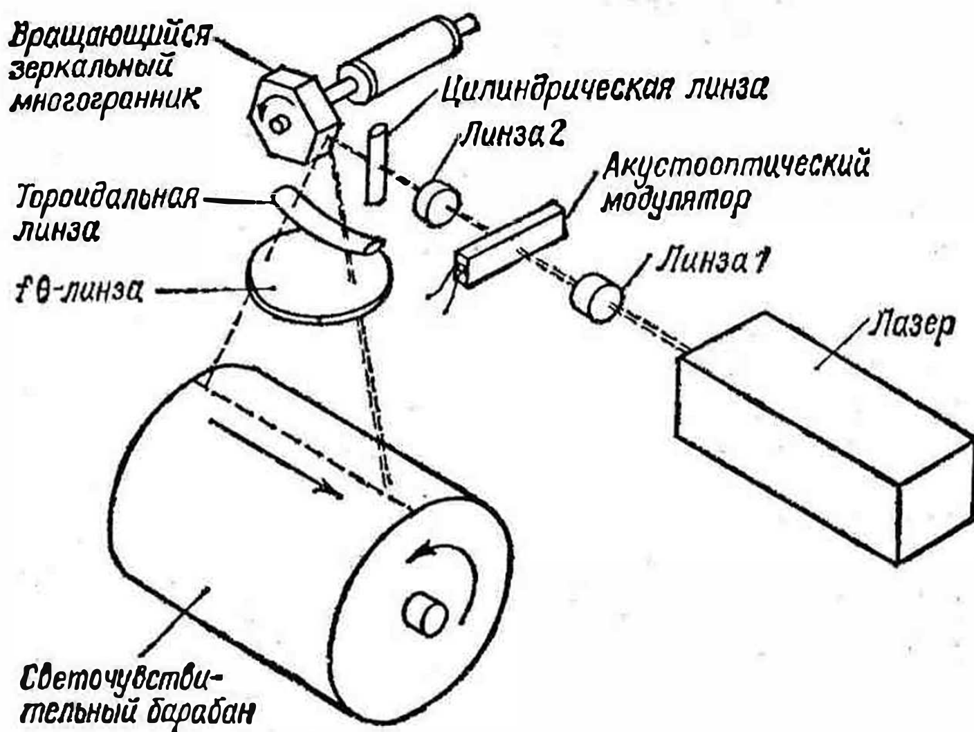
Рис. 137. Лазерная печать
