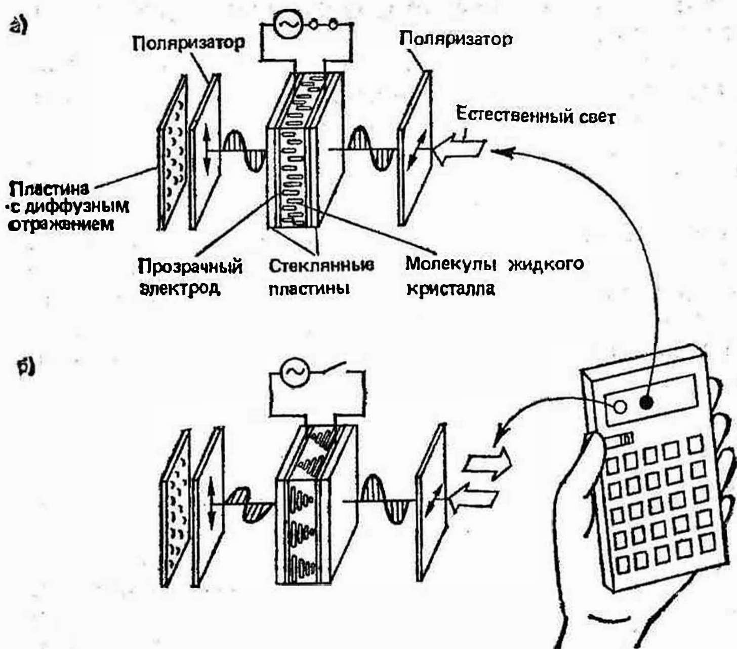
Рис. 70. Принцип действия пассивного дисплея: а — поглосение света (темное состояние); б — отражение света (светлое состояние)
