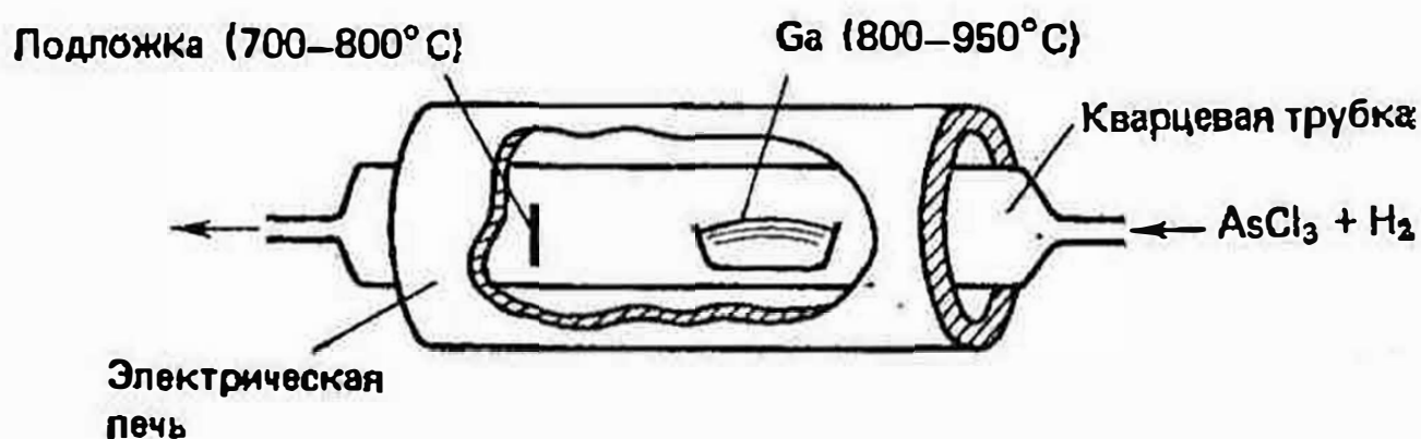
Рис. 42. Эпитаксия в газовой фазе
