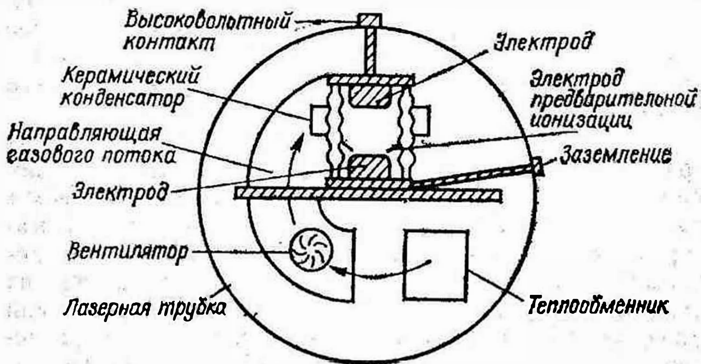
Рис. 63. Эксимерный лазер, возбуждаемый электрическим разрядом
