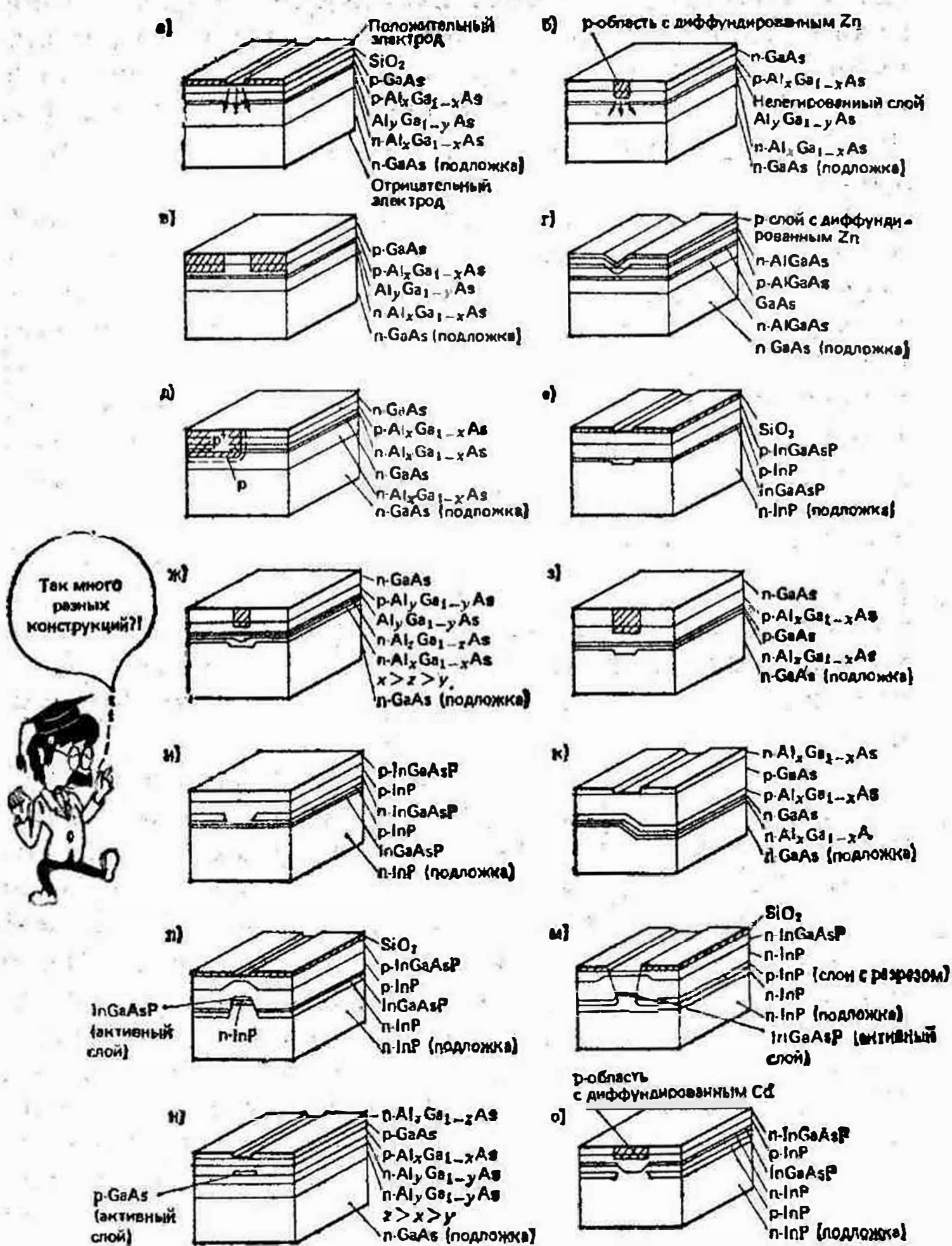
Рис. 53. Структуры полосковых лазеров: а — полоса SiO 2 ; б — полоса примеси; в — полоса, облученная пучком протонов; г — V-образная канавка; д — TJS-полоса (Transverse Junction Stripe); е — полоса в виде ребра; ж — PCW-полоса (Plano Complex Waveguide); з — CSP-полоса (Chanal Substrate Planar); и — самопроникающая полоса; к — TS-полоса (Terraced Substrate); л — врезанная полоса; м — ВН-полоса (Buried Hetero); н — SBH-полоса (Strip Buried Hetero); о — ВС-полоса (Buried Crescent)
