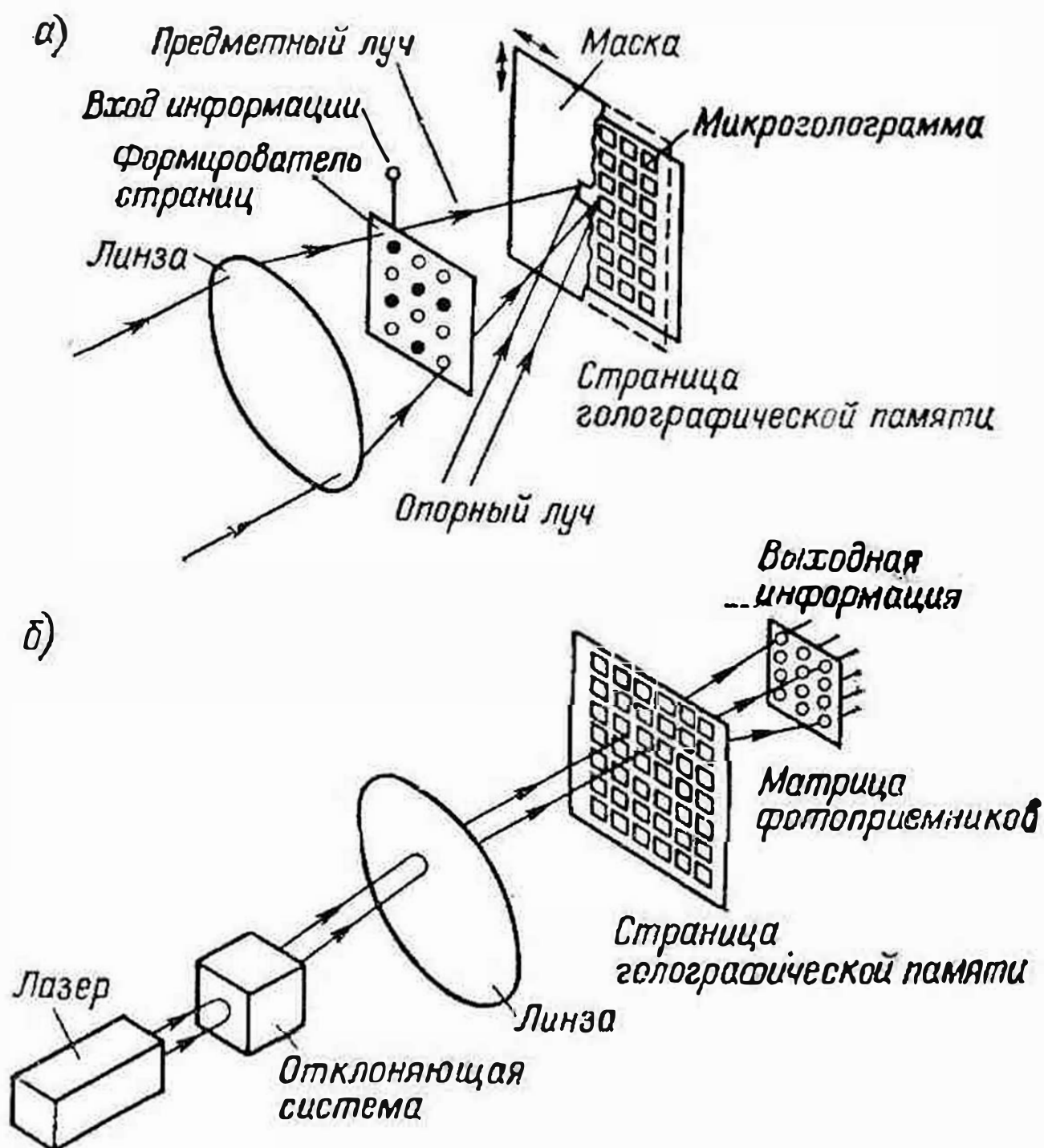
Рис. 117. Голографическая страничная память: а — запись; б — считывание
