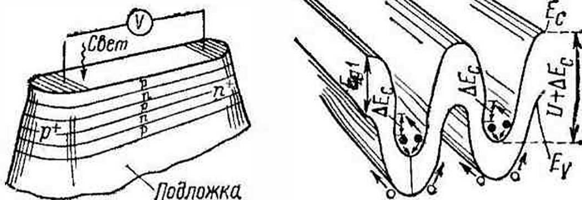
Рис. 121. Продольный лавинный фотодиод (F. Capasso, Electronics Letters, vol. 18, No. 1, p. 12, 1982)
