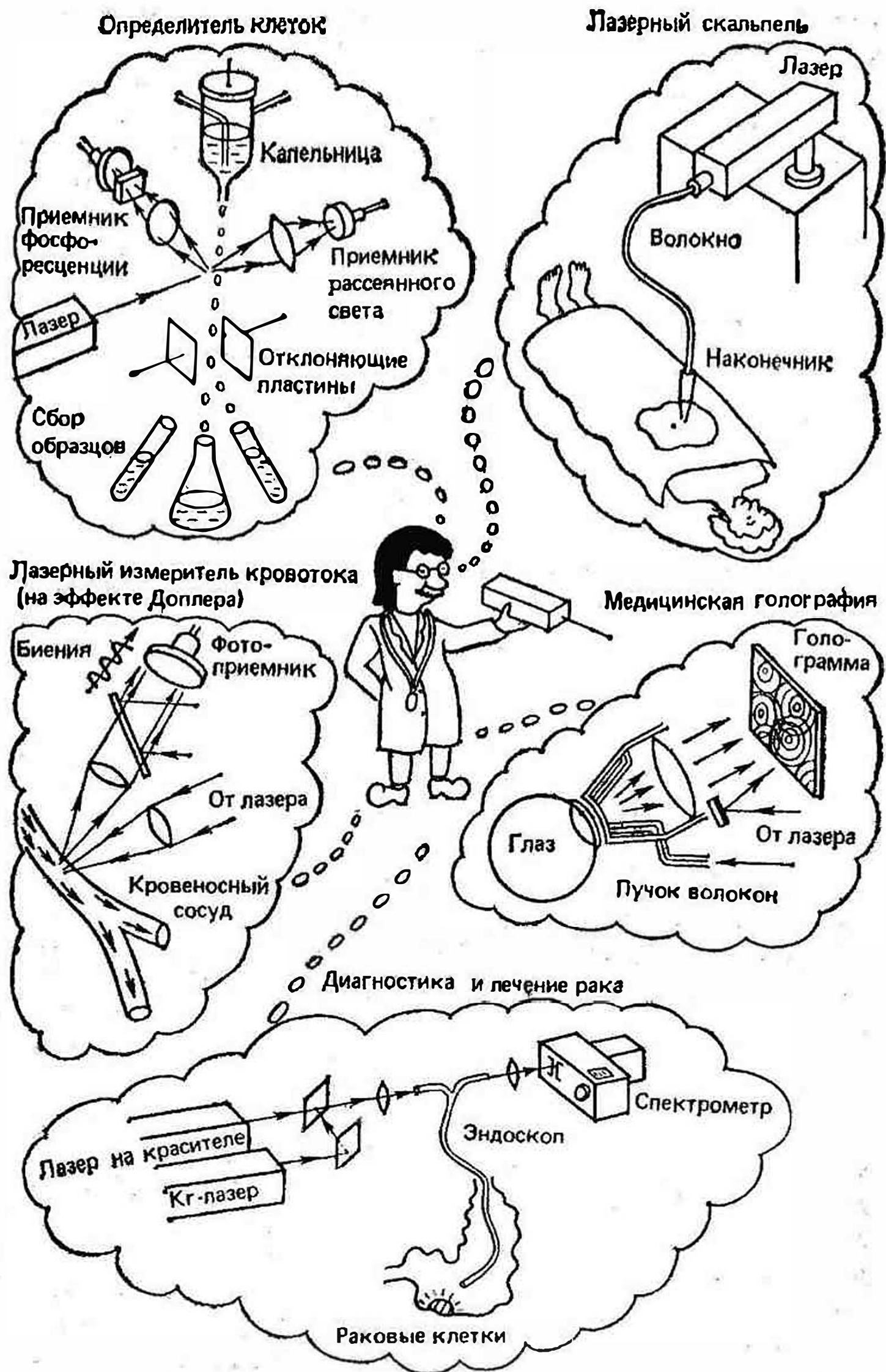
Рис. 135. Приборы лазерной медицины
