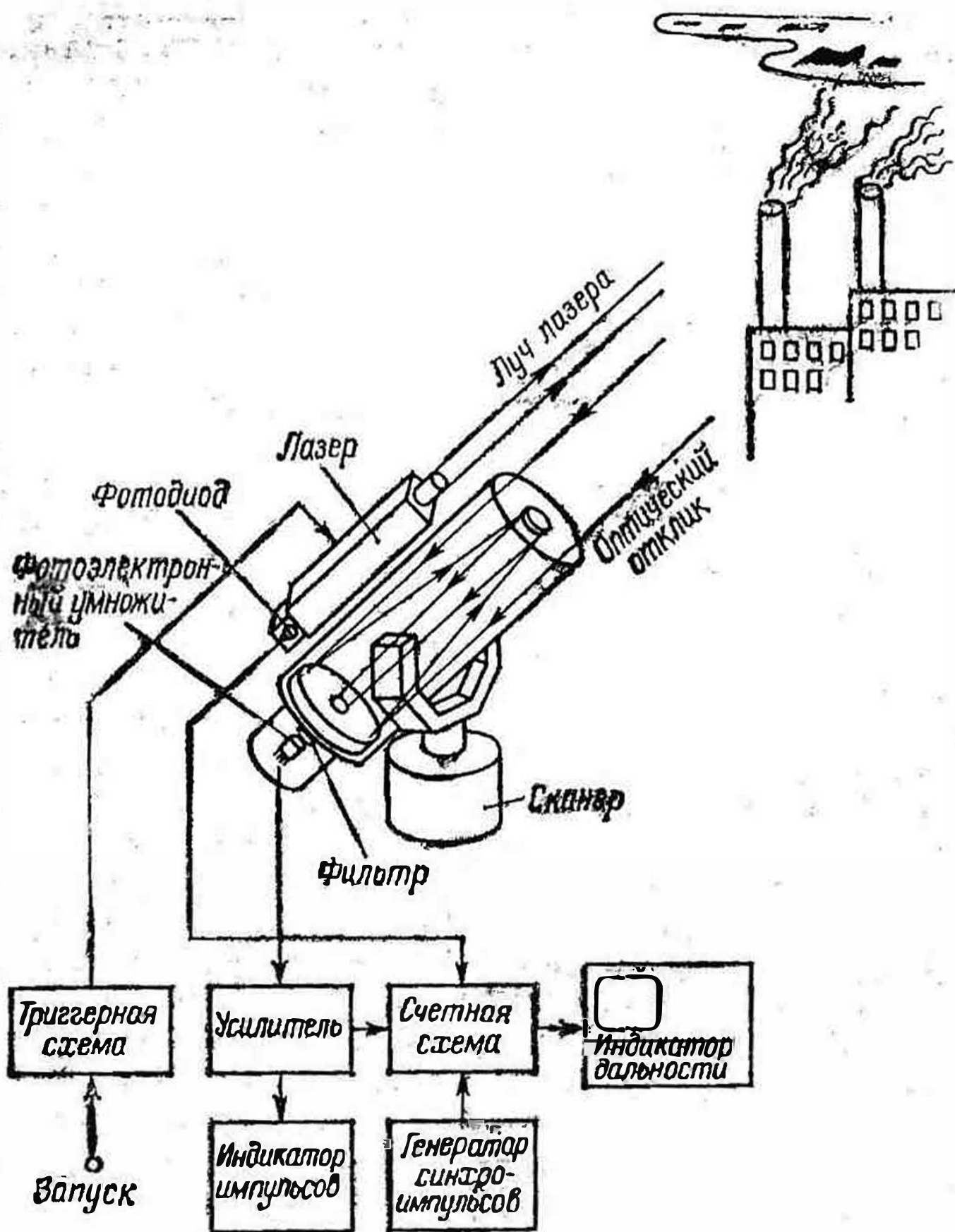
Рис. 130. Лазерный радар
