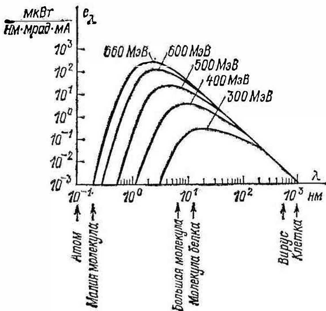
Рис. 8. Спектр синхротронного излучения
