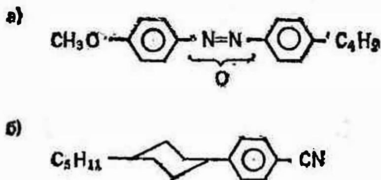
Рис. 78. Структурные формулы: а — 4-бутил-4'-метоксиназоксикарбонилбензол; б — 1-(транс-4'-пентилциклогексил)-4-цианобензол
