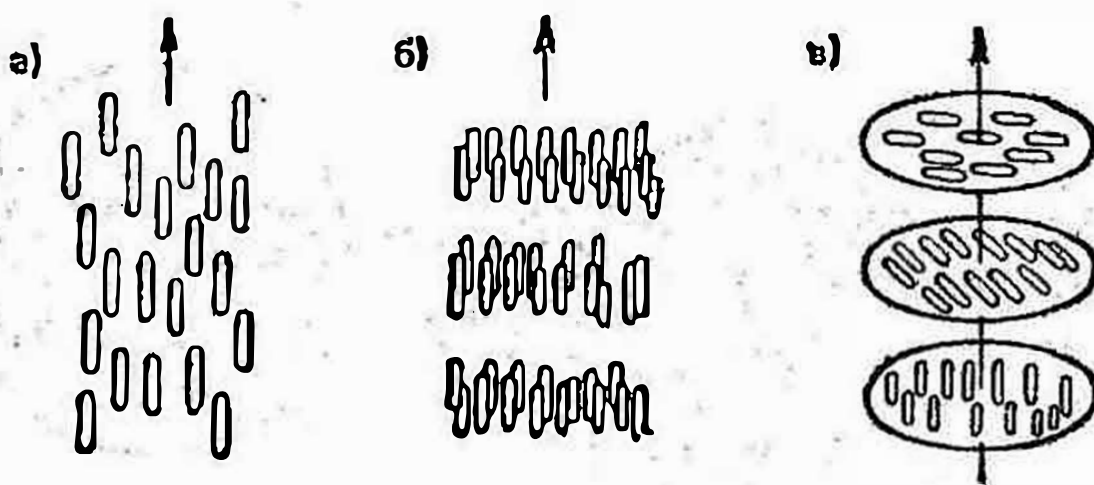
Рис. 77. Расположение молекул в жидких кристаллах: а — нематическое; б — смектическое; в — холестерическое
