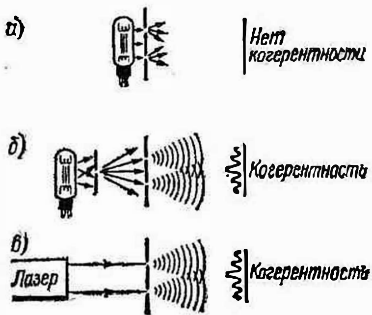
Рис. 14. Наблюдение пространственной когерентности на двух щелях
