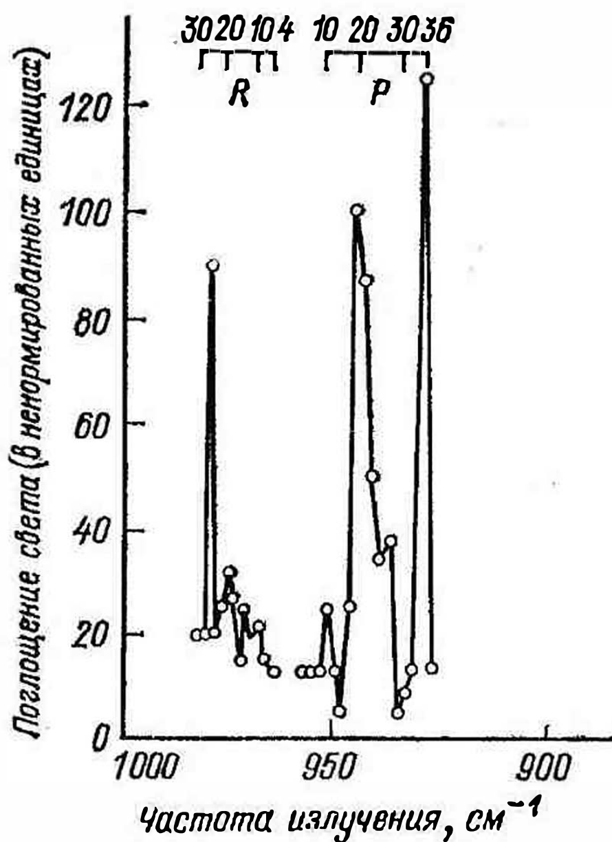
Рис. 48. Поглощение света моносиланом с возбуждением колебательных уровней
