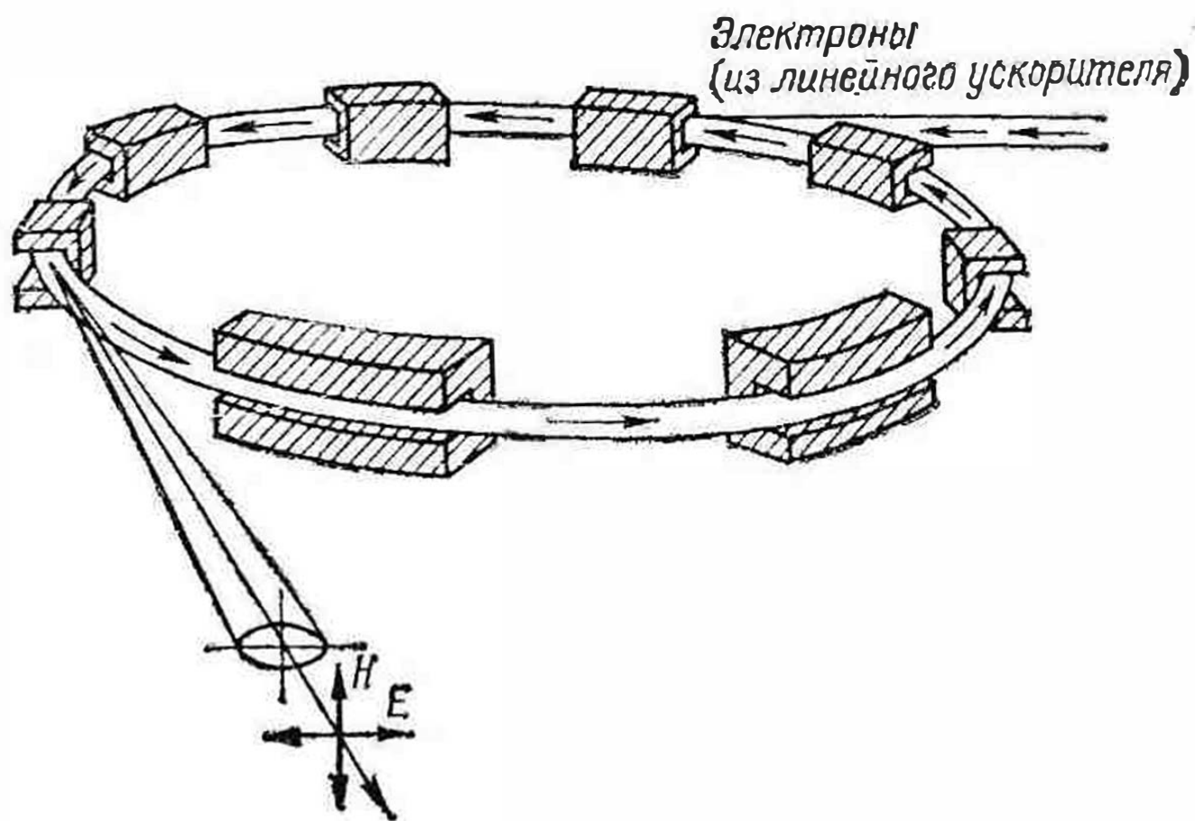
Рис. 7. Схема возникновения синхротронного излучения
