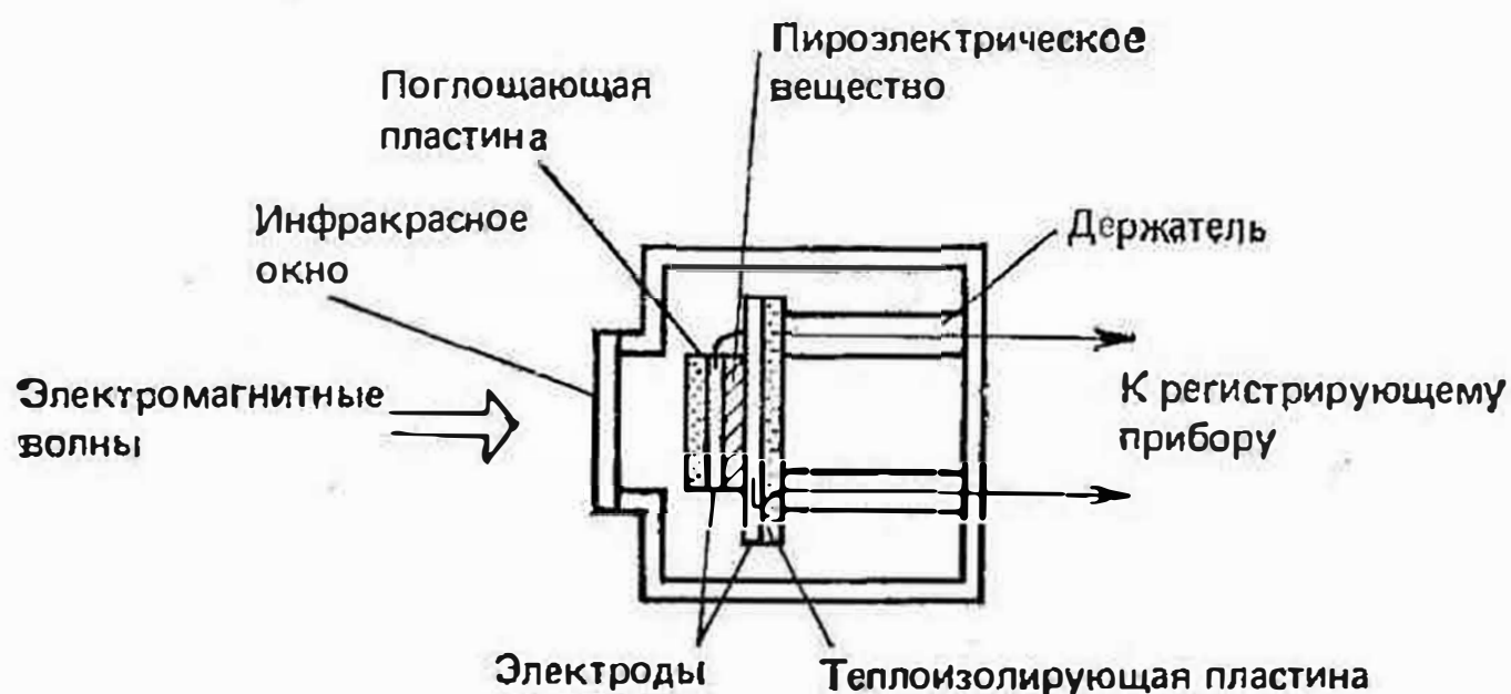
Рис. 34. Пироэлектрический датчик
