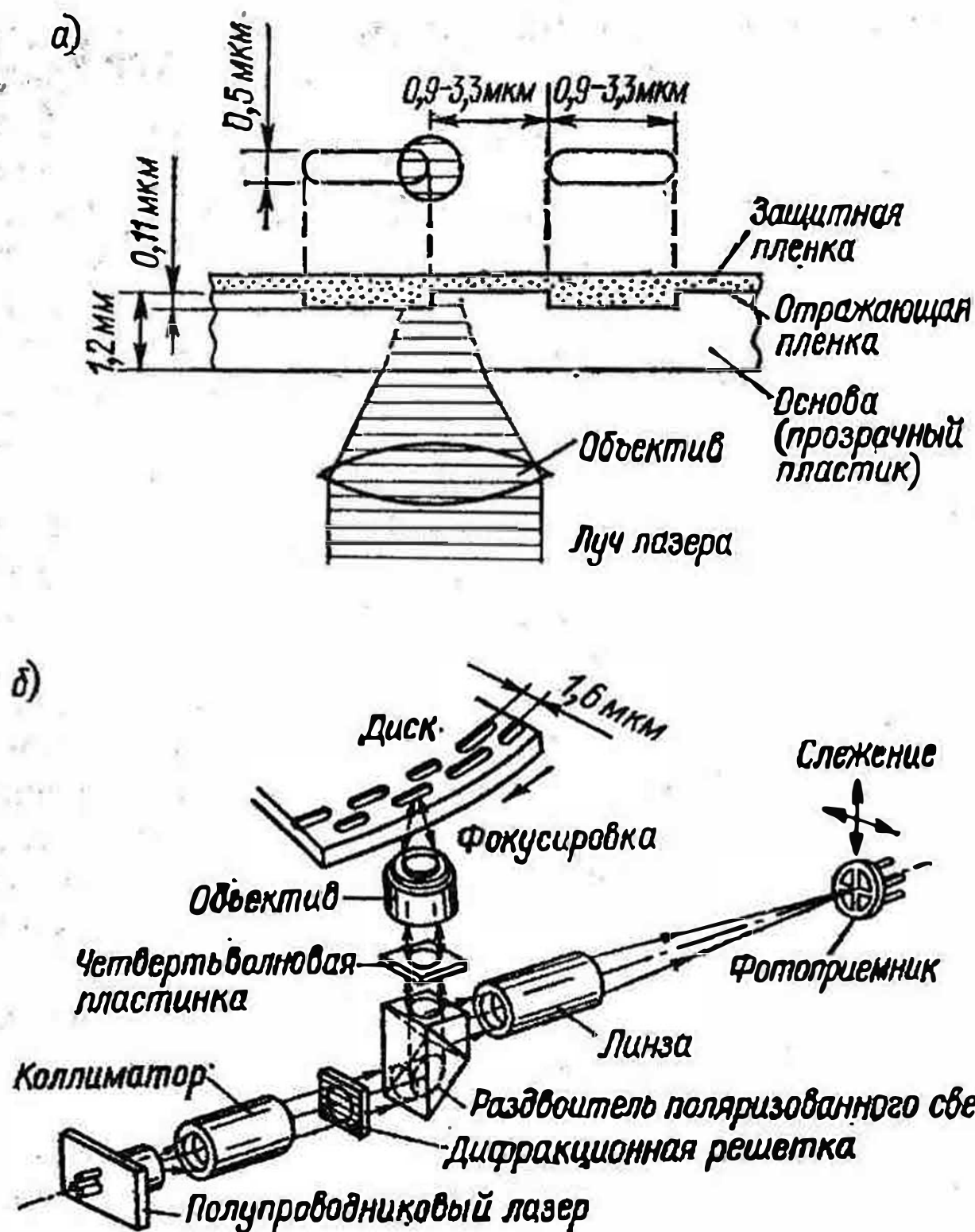
Рис. 129. Принцип устройства и работы оптического диска
