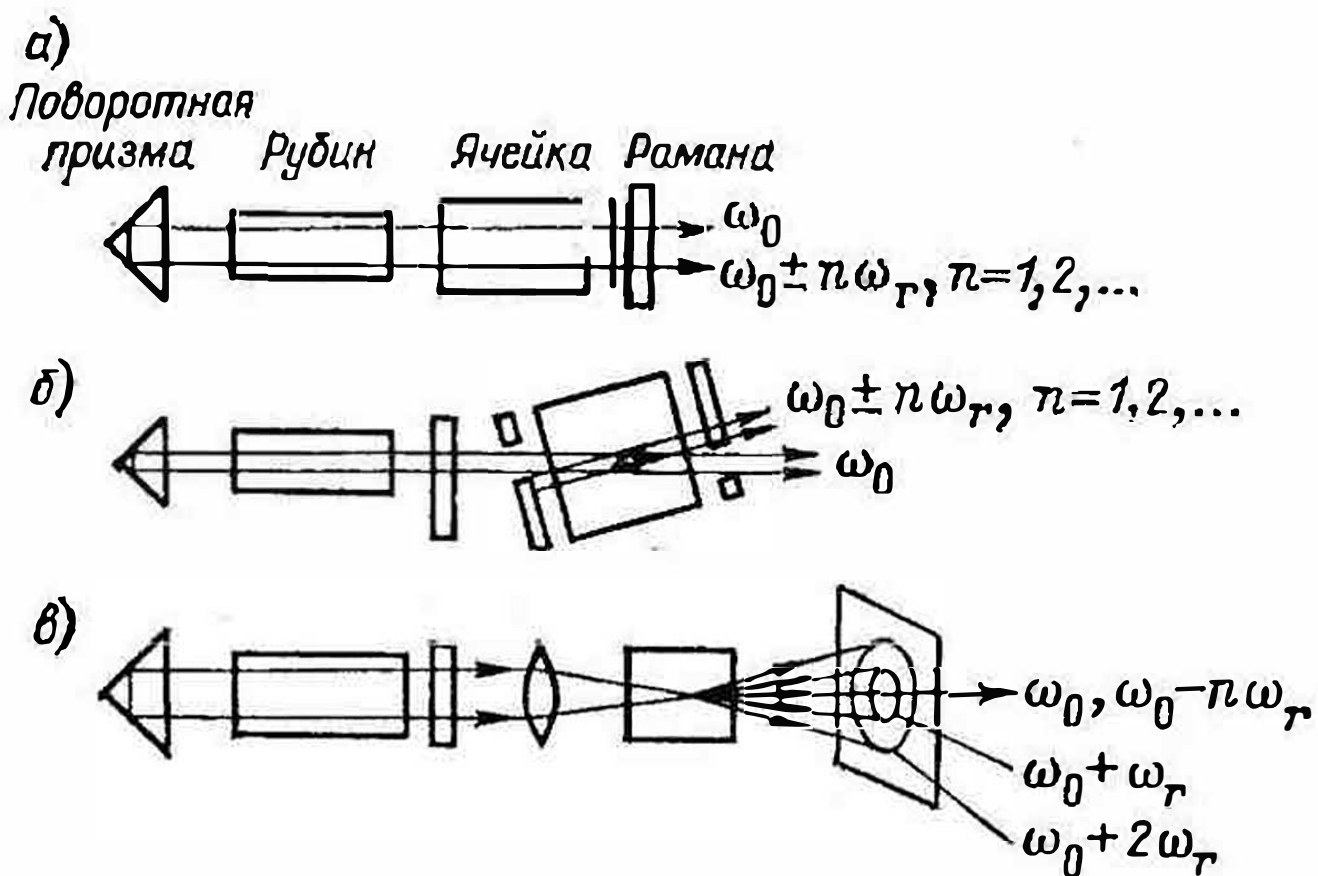
Рис. 23. Различные виды рамановских лазеров
