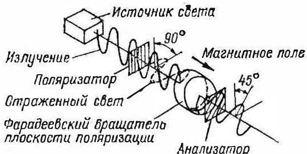
Рис. 106. Принцип работы оптического вентиля
