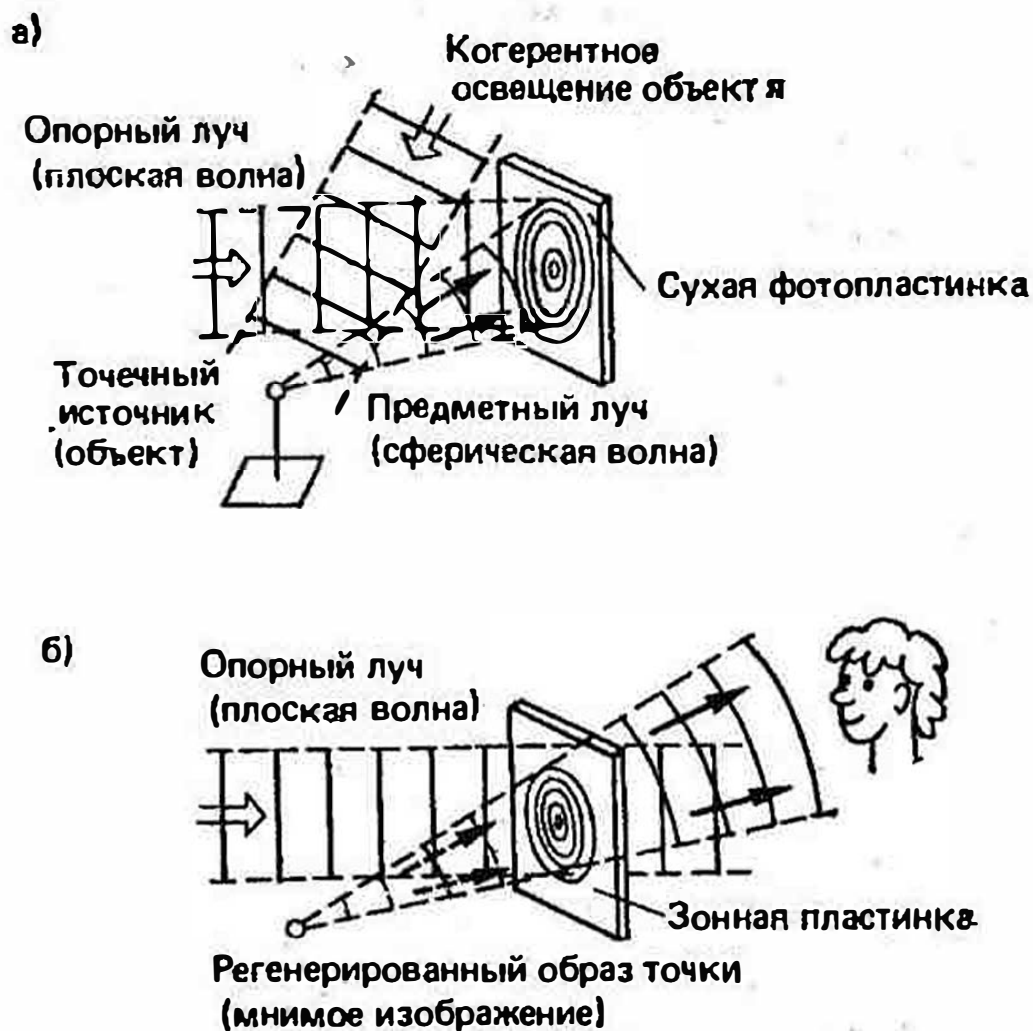
Рис. 127. Принцип голографин: а — получение зонной пластинки; б — регенерация изображения с зонной пластинки
