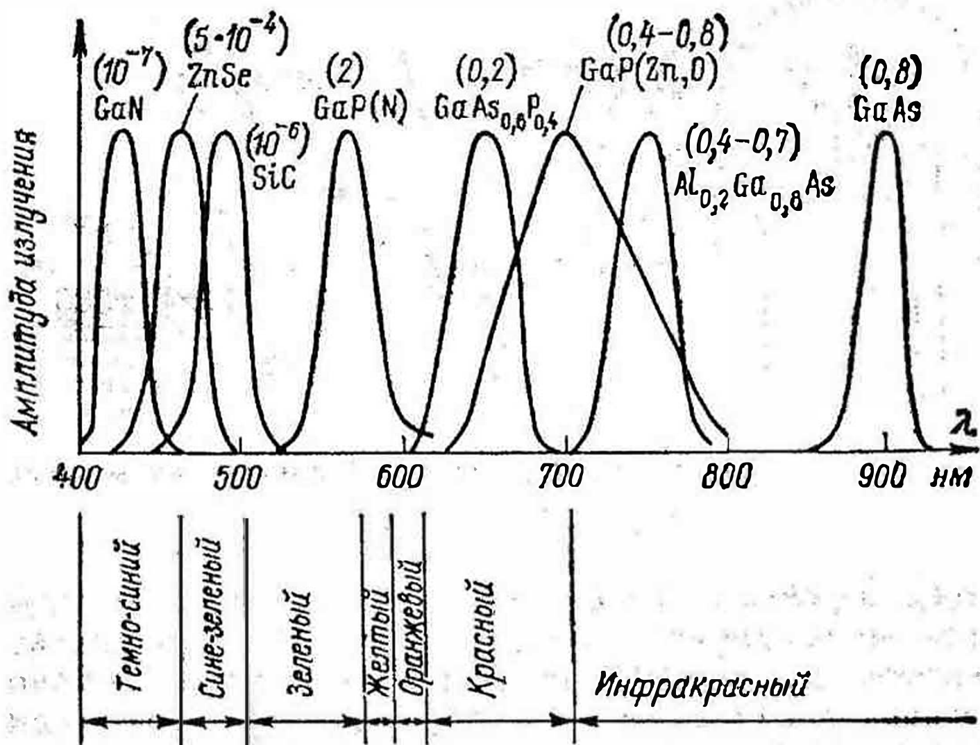
Рис. 73. Спектры излучения светодиодов.
