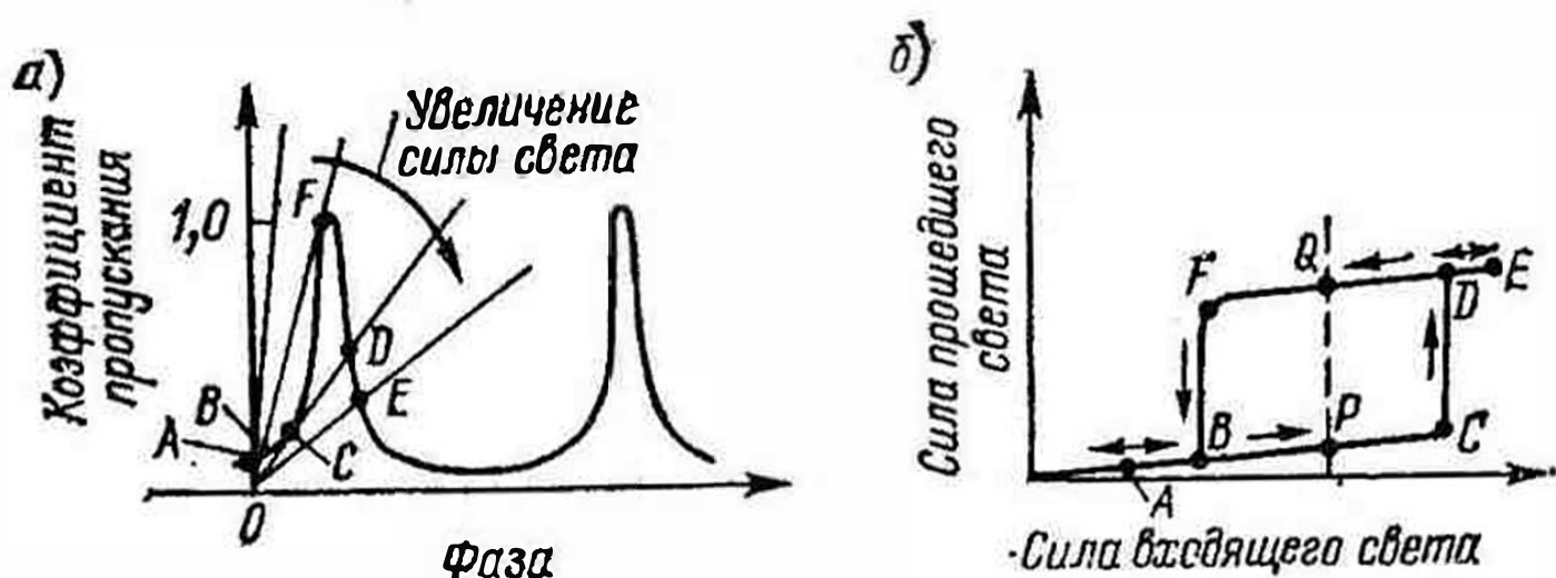
Рис. 102. Характеристики оптического бистабильного элемента: а — нагрузочная; б — круглая гистерезиса
