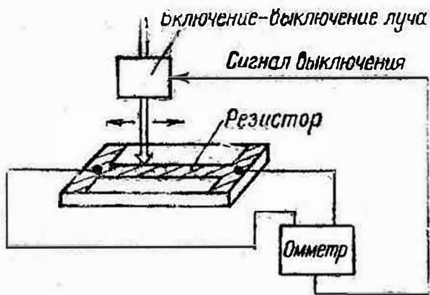
Рис. 134. Лазерная доводка
