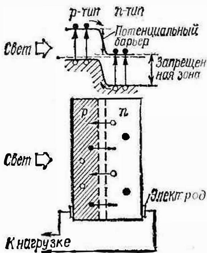
Рис. 90. Структура и диаграмма энергетических уровней солнечной батареи
