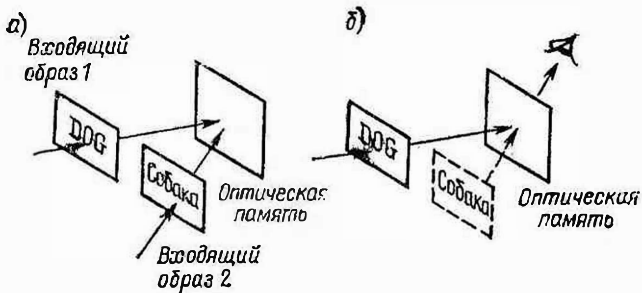
Рис. 118. Функциональная голографическая память: а — запись; б — считывание
