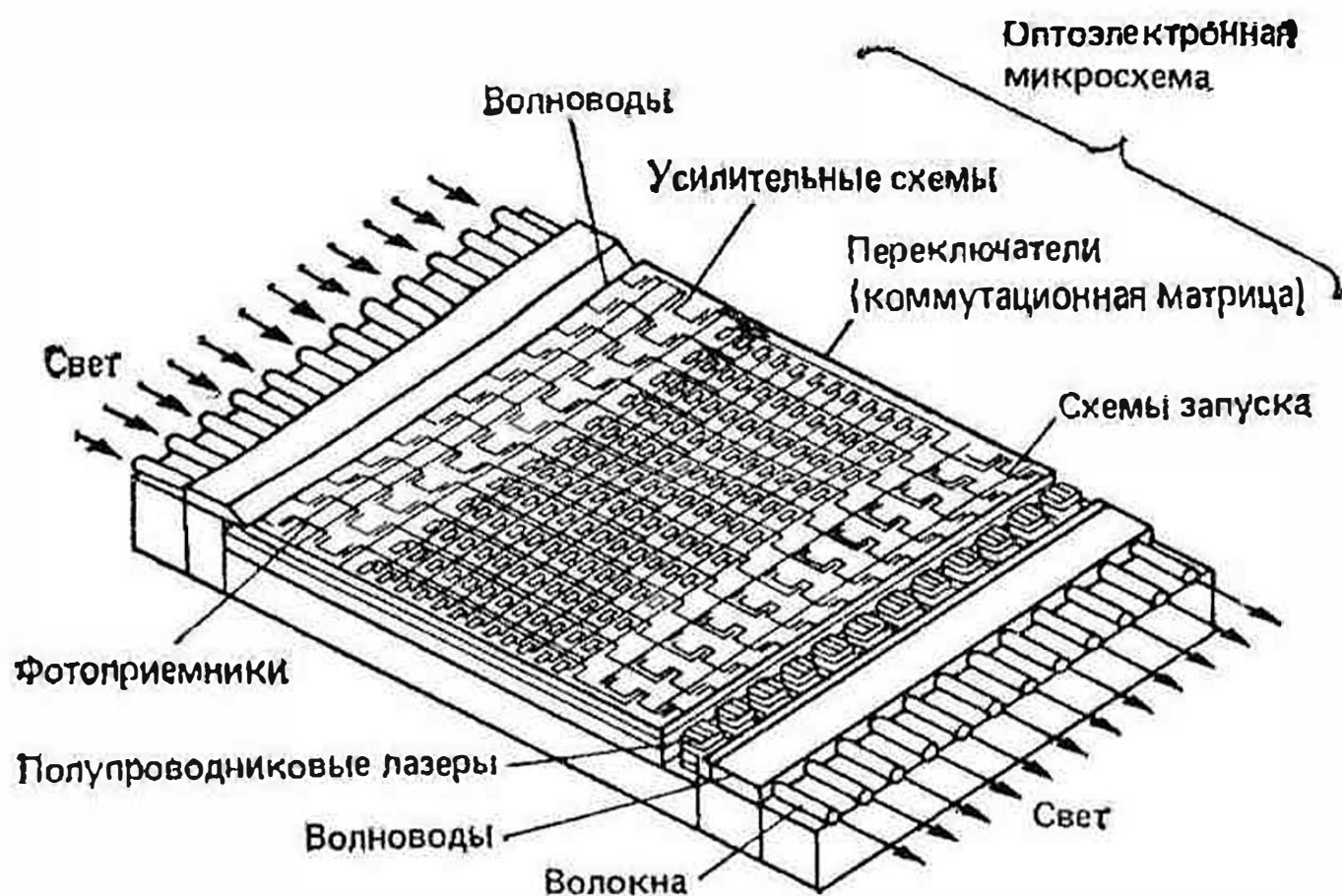
Рис. 120. Оптоэлектронная интегральная схема — многоканальный ретранслятор
