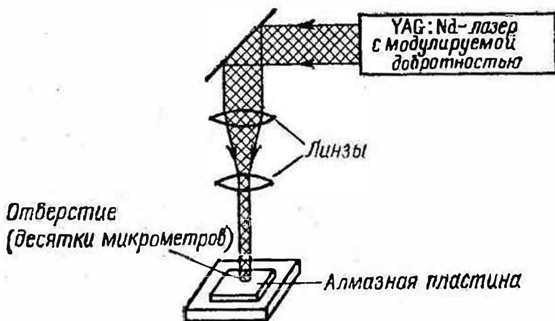
Рис. 133. Лазерное сверление
