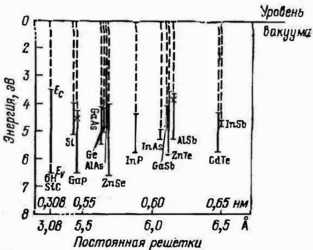
Рис. 41. Сродство к электрону (штриховая линия), ширина запрещенной зоны (сплошная линия) и постоянная решетки различных полупроводников
