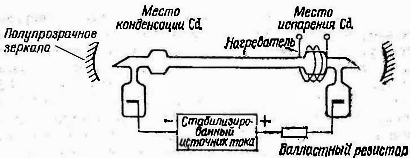
Рис. 60. Гелий-кадмиевый лазер
