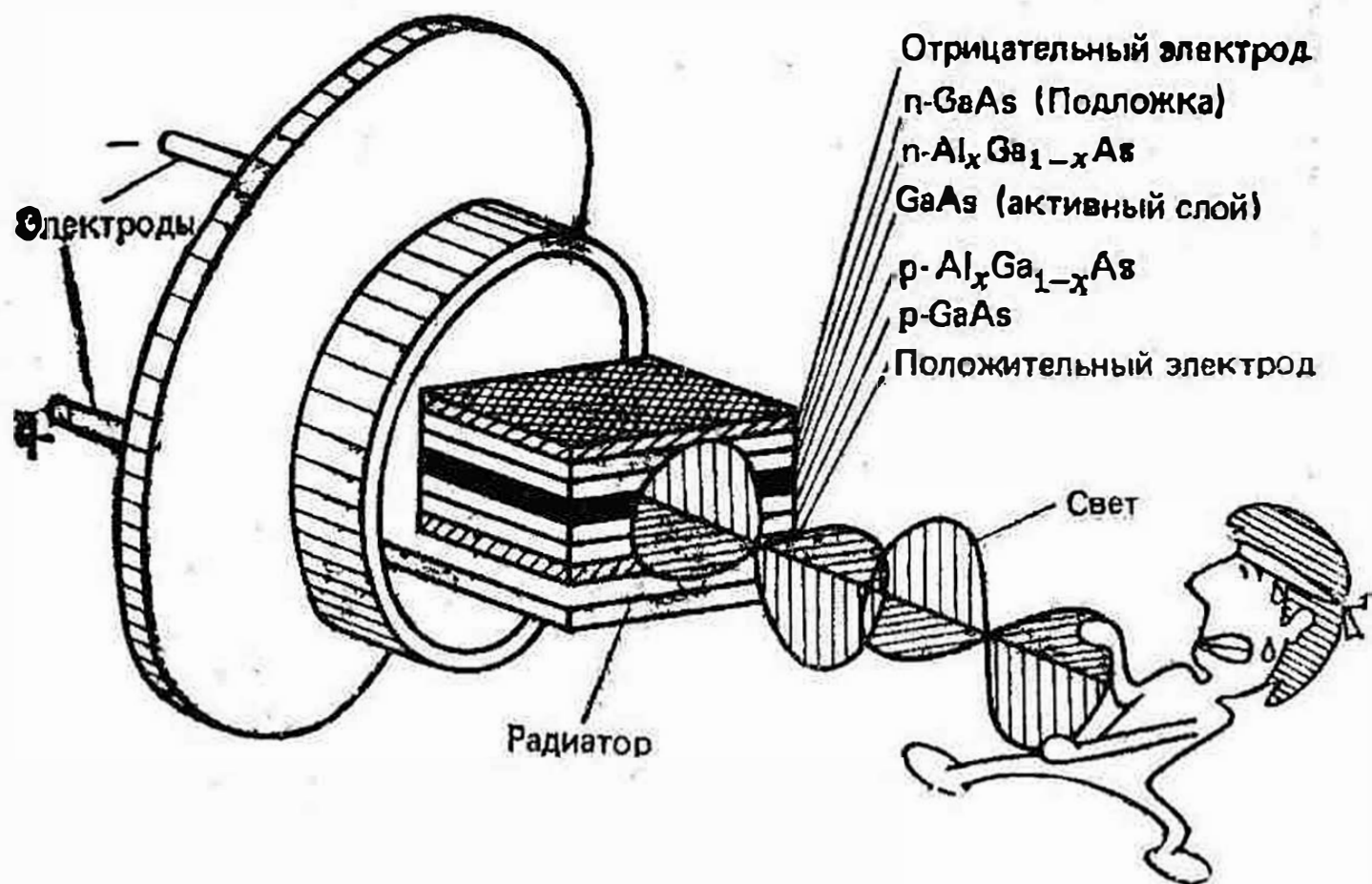
Рис. 51. Полупроводниковый лазер
