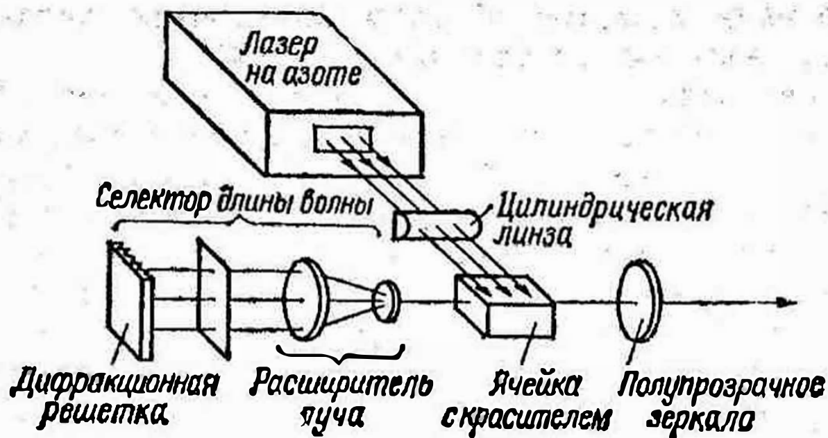
Рис. 68. Лазер на красителе, возбуждаемый излучением азотного лазера
