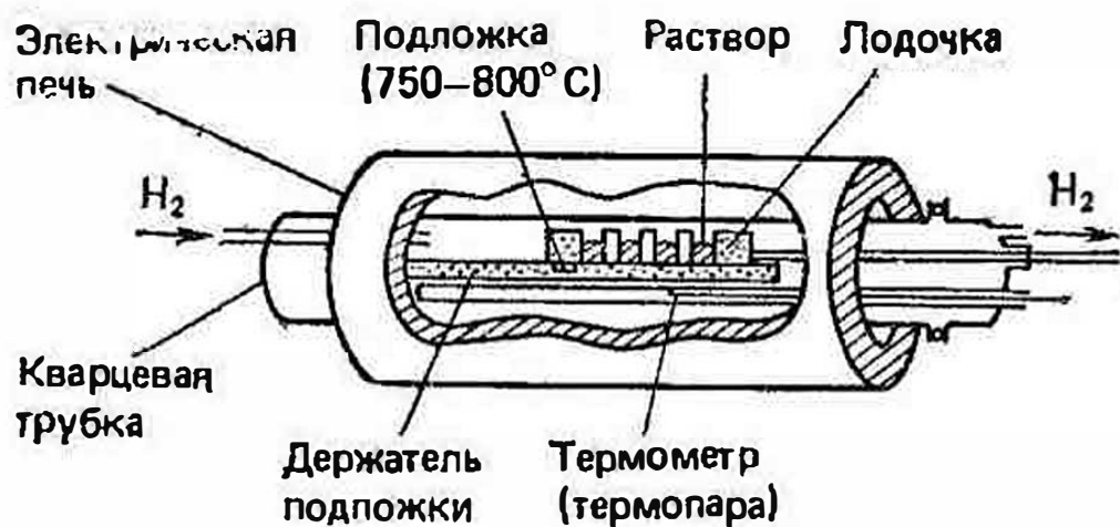
Рис. 44. Эпитаксия в жидкой фазе
