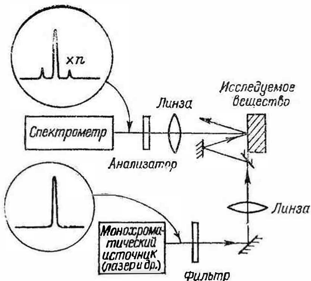
Рис. 21. Система для наблюдения эффекта Рамана
