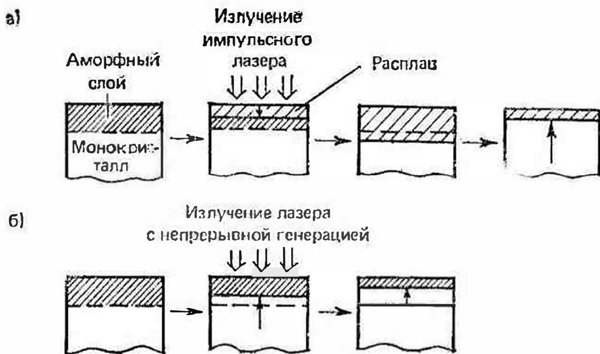
Рис. 49. Отжиг импульсным лазером (а) и лазером с непрерывной генерацией (б)
