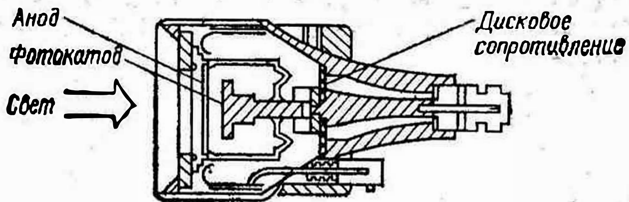
Рис. 81. Бипланарный фотоэлемент
