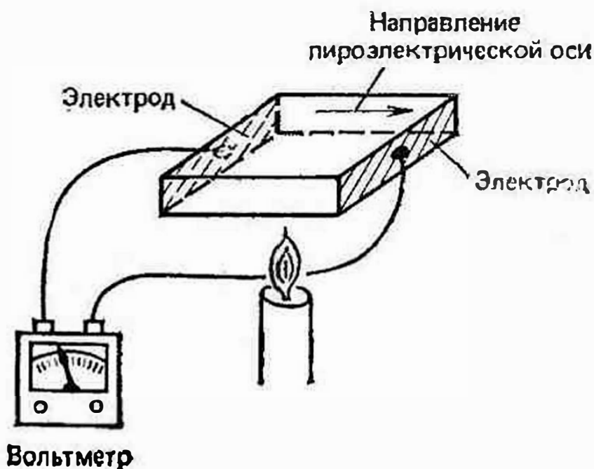
Рис. 32. Наблюдение пироэлектрического эффекта
