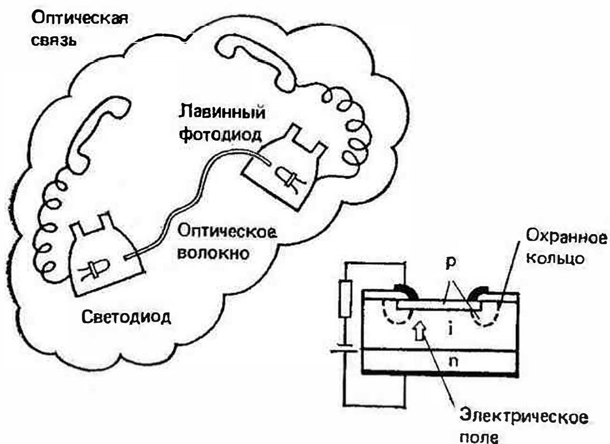
Рис. 86. Лавинный фотодиод
