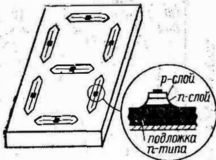
Рис. 72. Светодиодная матрица
