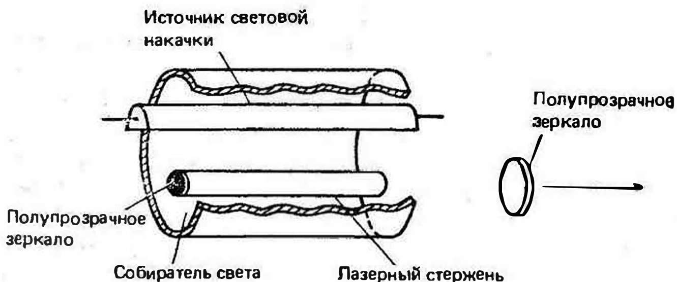
Рис. 64. Твердотельный лазер
