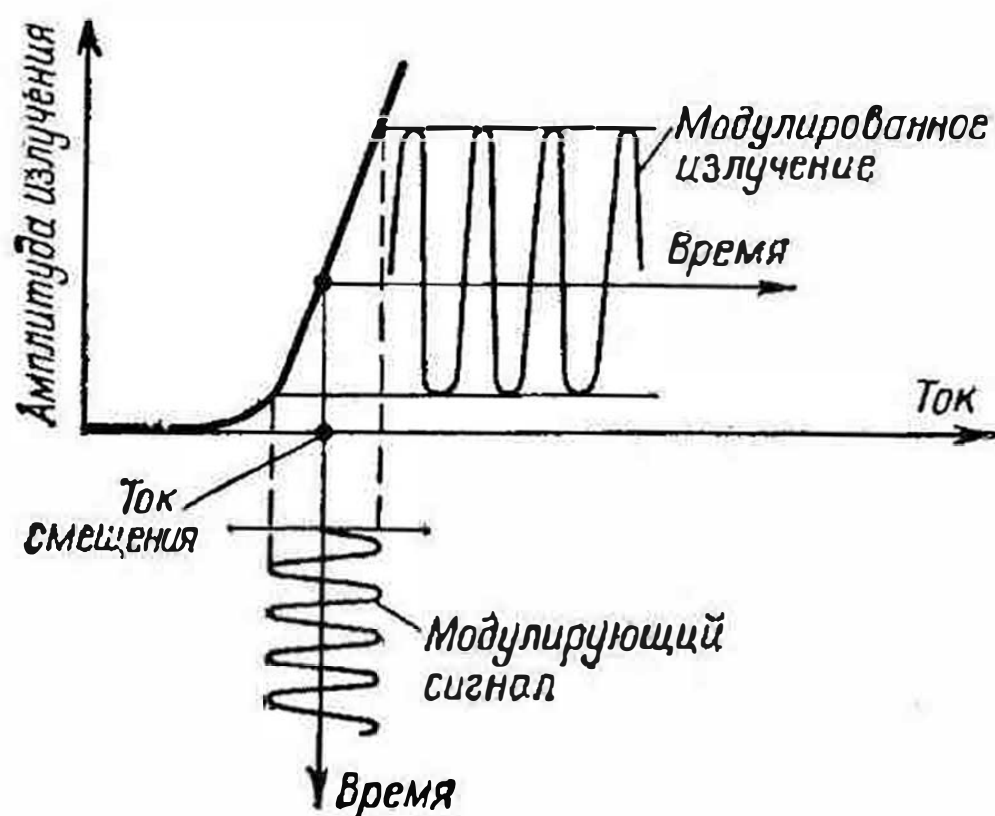
Рис. 98. Непосредственная модуляция в полупроводниковом лазере
