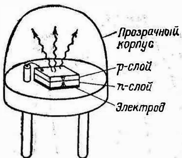
Рис. 71. Светодиод
