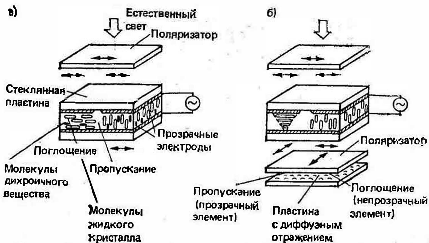
Рис. 79. Дисплеи на жидких кристаллах
