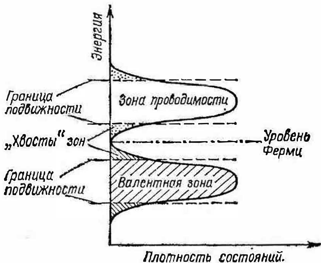
Рис. 38. Зонная структура аморфного полупроводника
