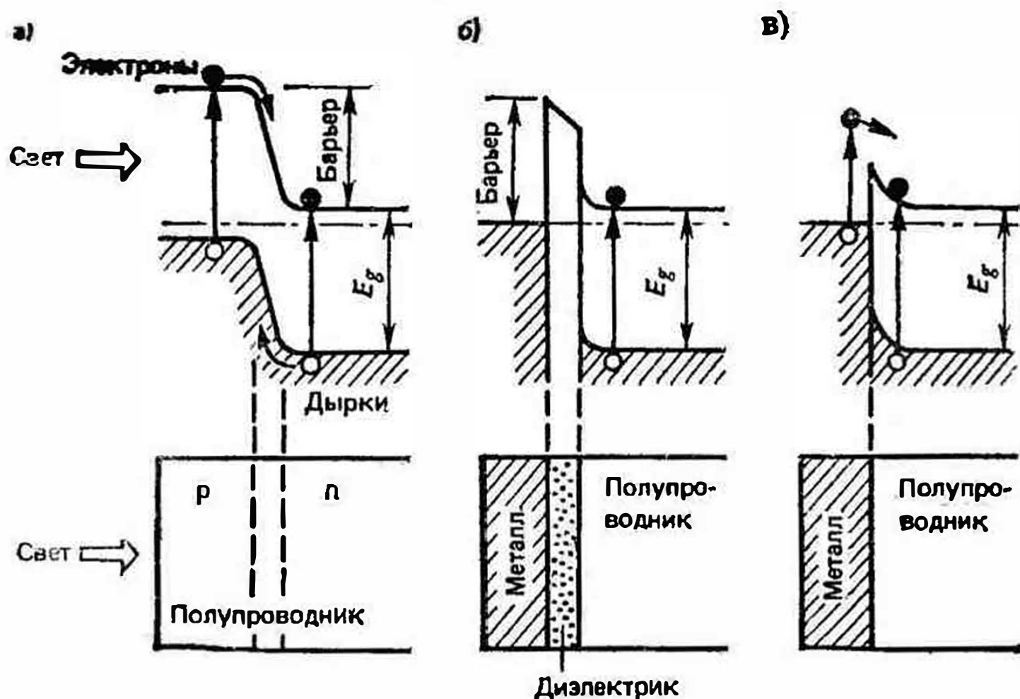
Рис. 31. Механизм барьерного фотоэффекта
