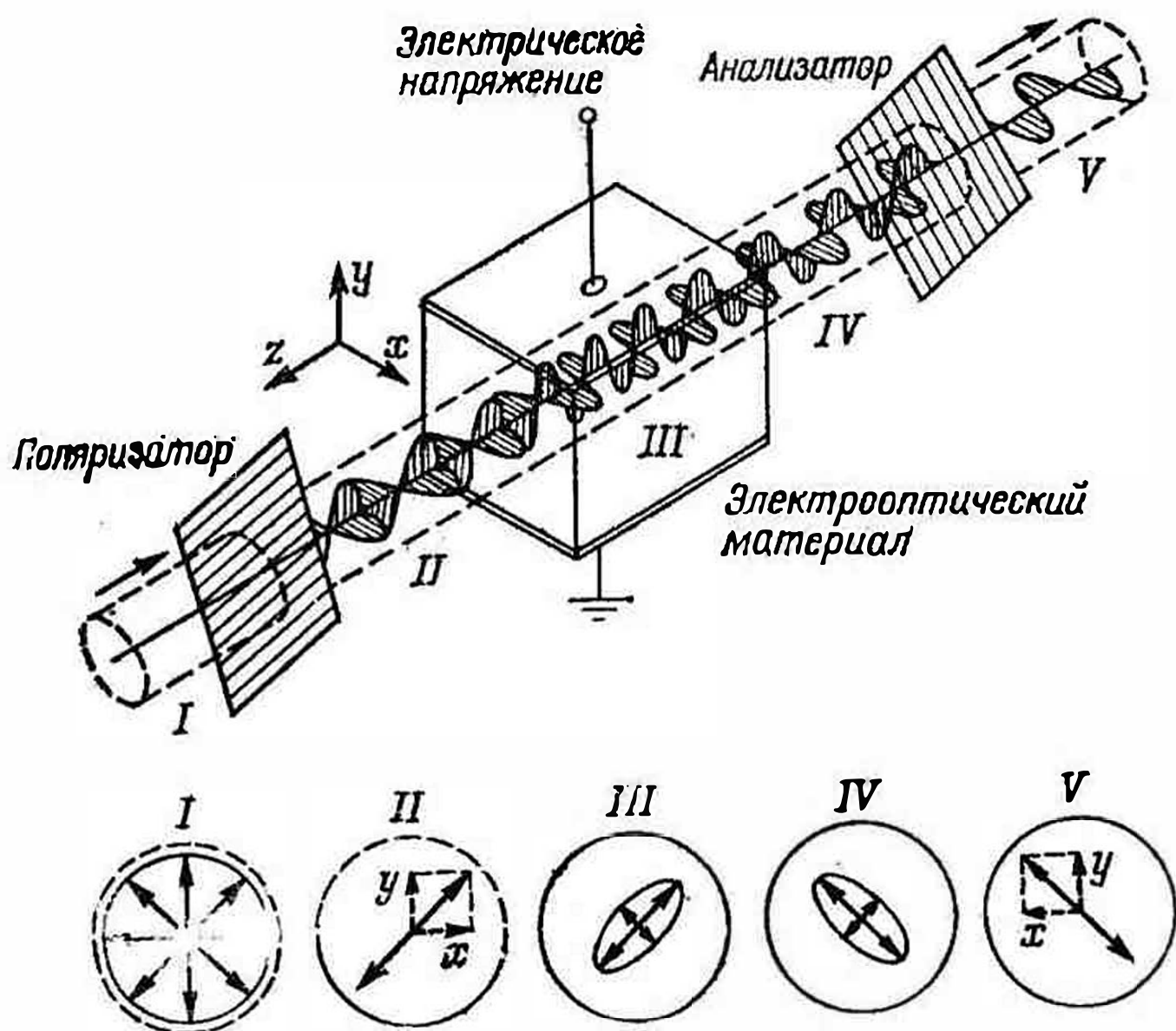
Рис. 15. Модуляция света на основе электрооптического эффекта Поккельса
