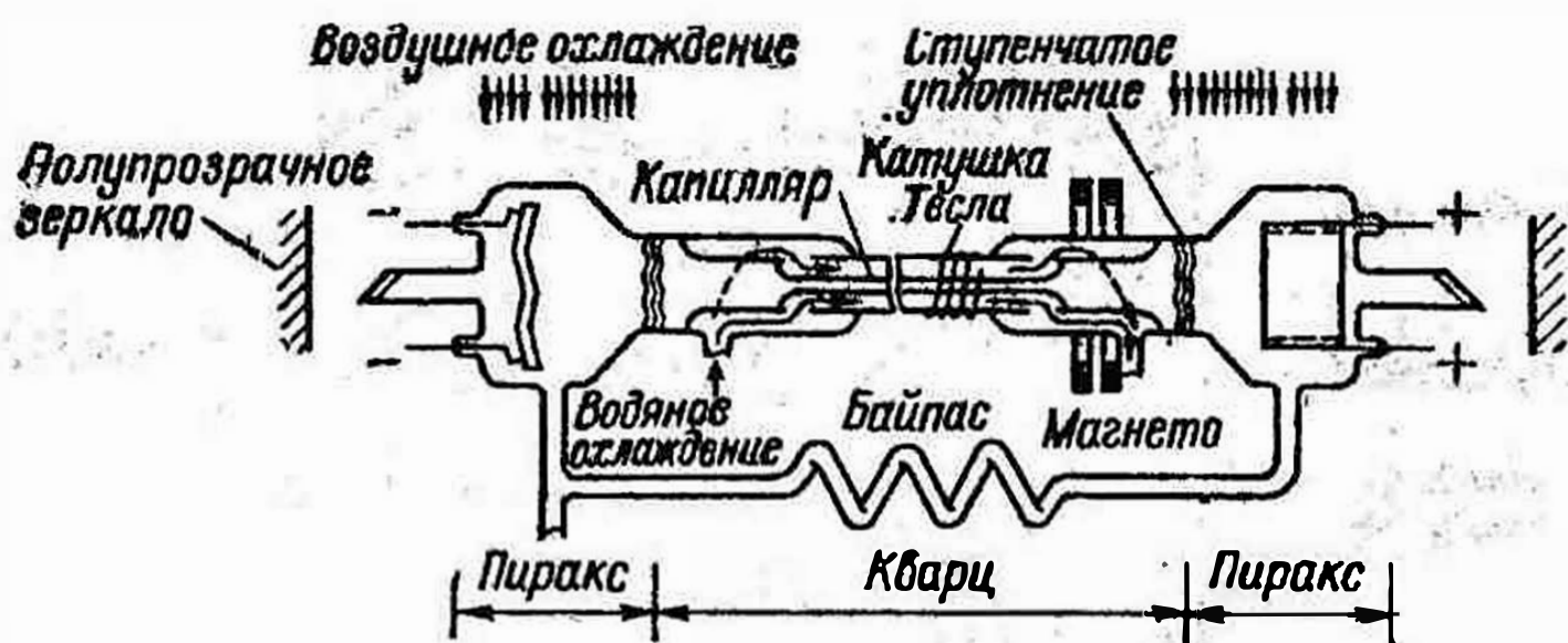
Рис. 59. Аргоновый лазер
