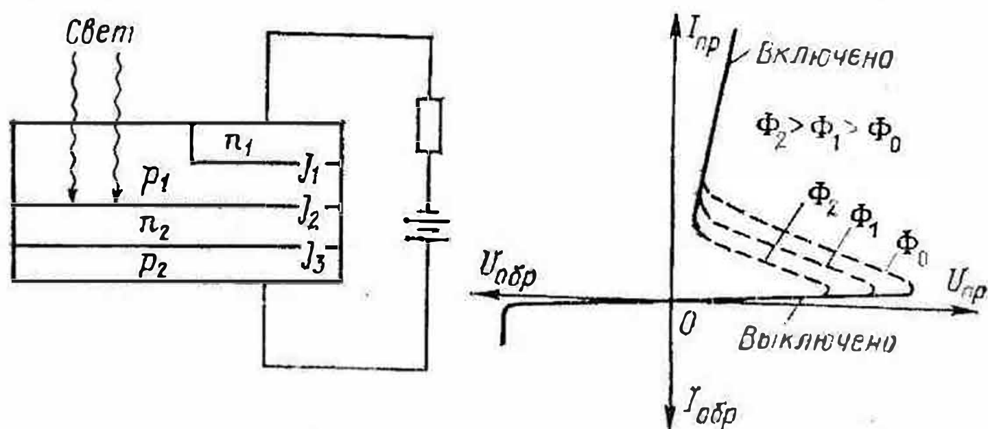
Рис. 88. Устройство и вольт-амперная характеристика фототиристора
