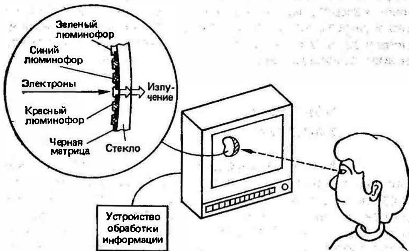
Рис. 69. Цветной дисплей на трубке Брауна
