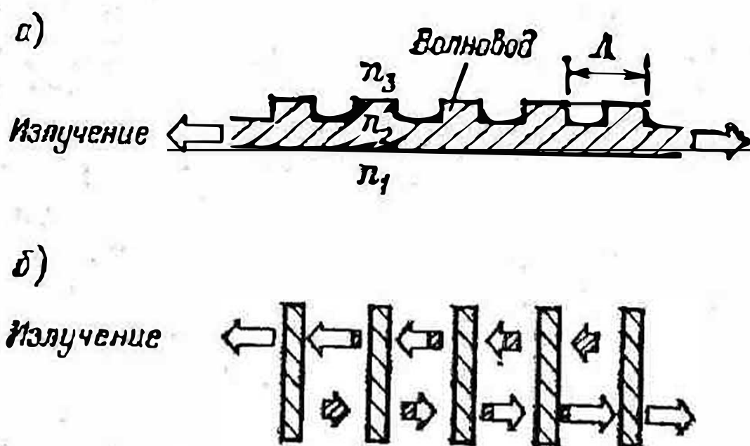
Рис. 54. Лазерная генерация в волноводе с периодической структурой
