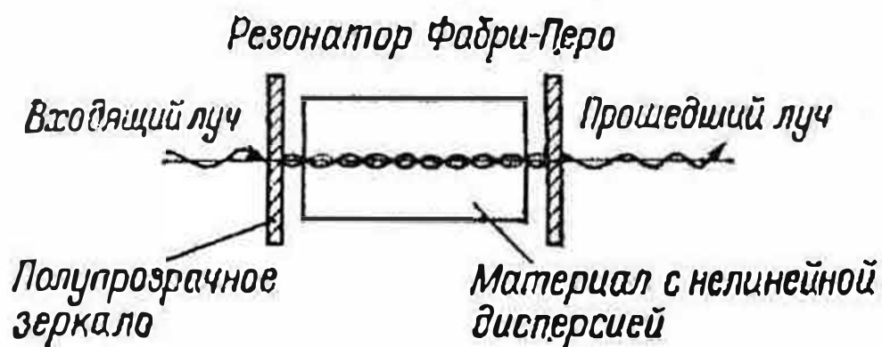
Рис. 101. Оптический бистабильный элемент
