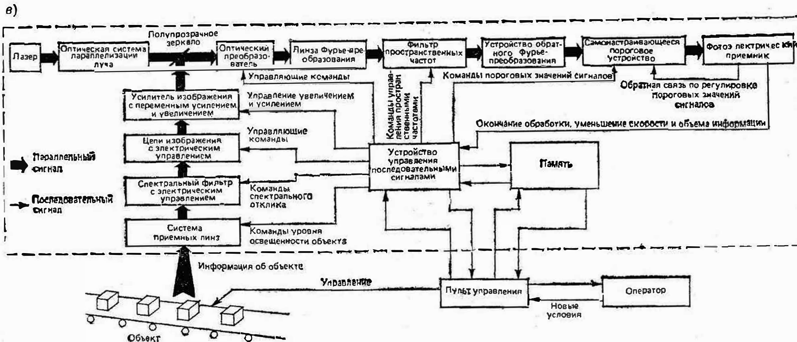
Рис. 126. Принцип последовательной (а), параллельной цифровой (б) и параллельной аналоговой (в) обработки в оптическом компьютере
