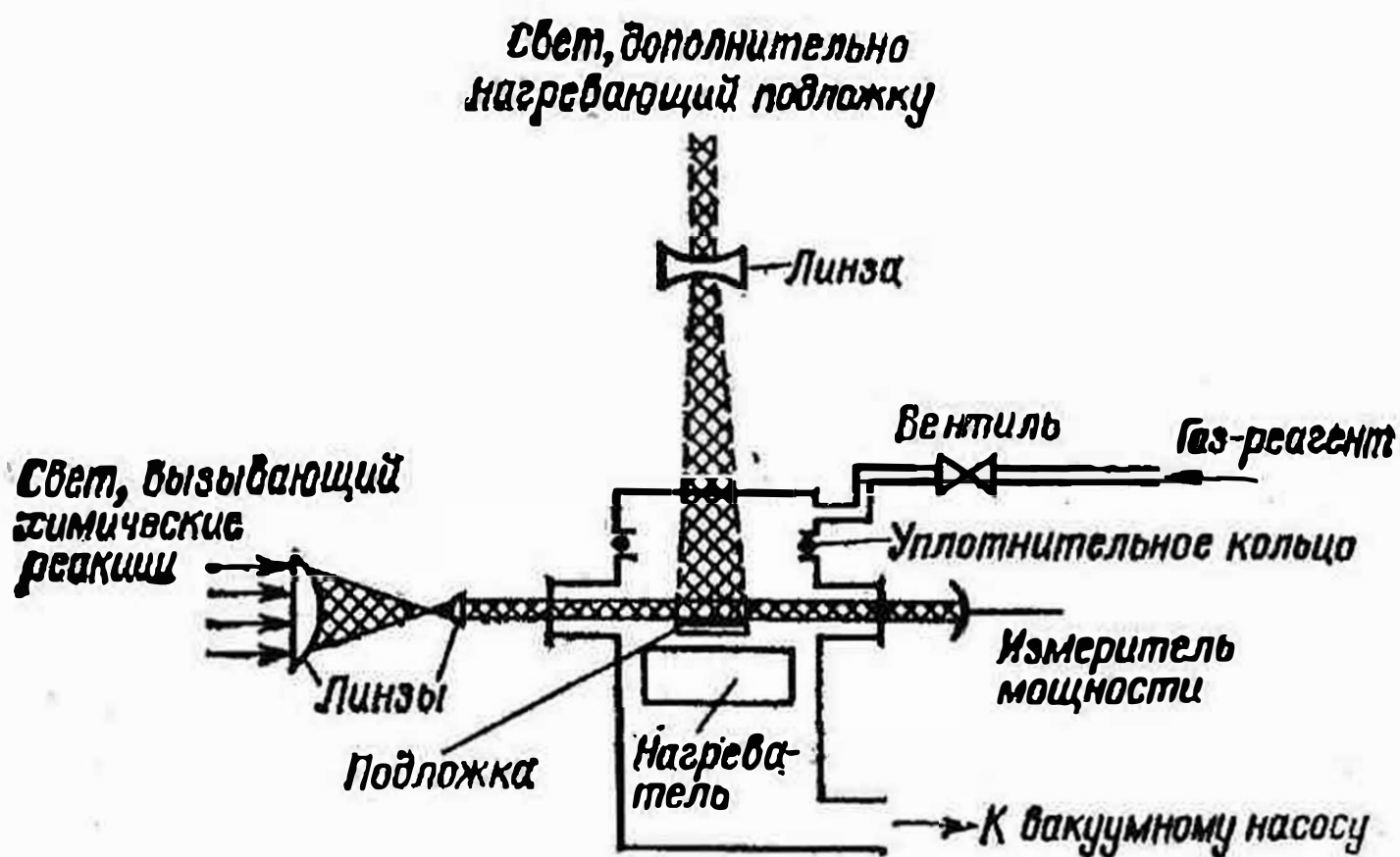
Рис. 47. Химическое осаждение с помощью света
