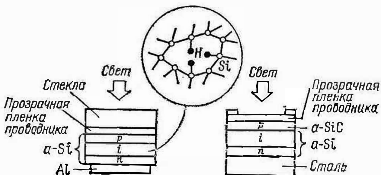
Рис. 92. Солнечный элемент на аморфном кремнии ( \alpha = \text{Si} ) Слева p-i-n -структура на стекле (в круге показаны свободные связи водорода и кремния); справа p-i-n -структура на стали с окном из карбида кремния, имеющего широкую запрещенную зону
