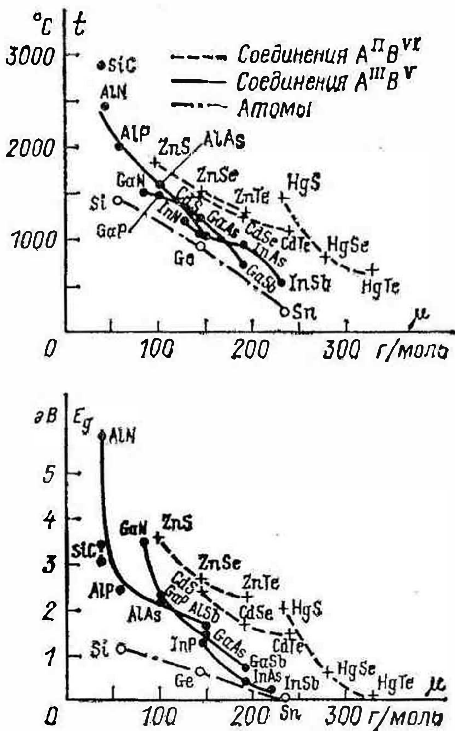
Рис. 36. Температура плавления и ширина запрещенной зоны полупроводниковых соединений в зависимости от молярной массы
