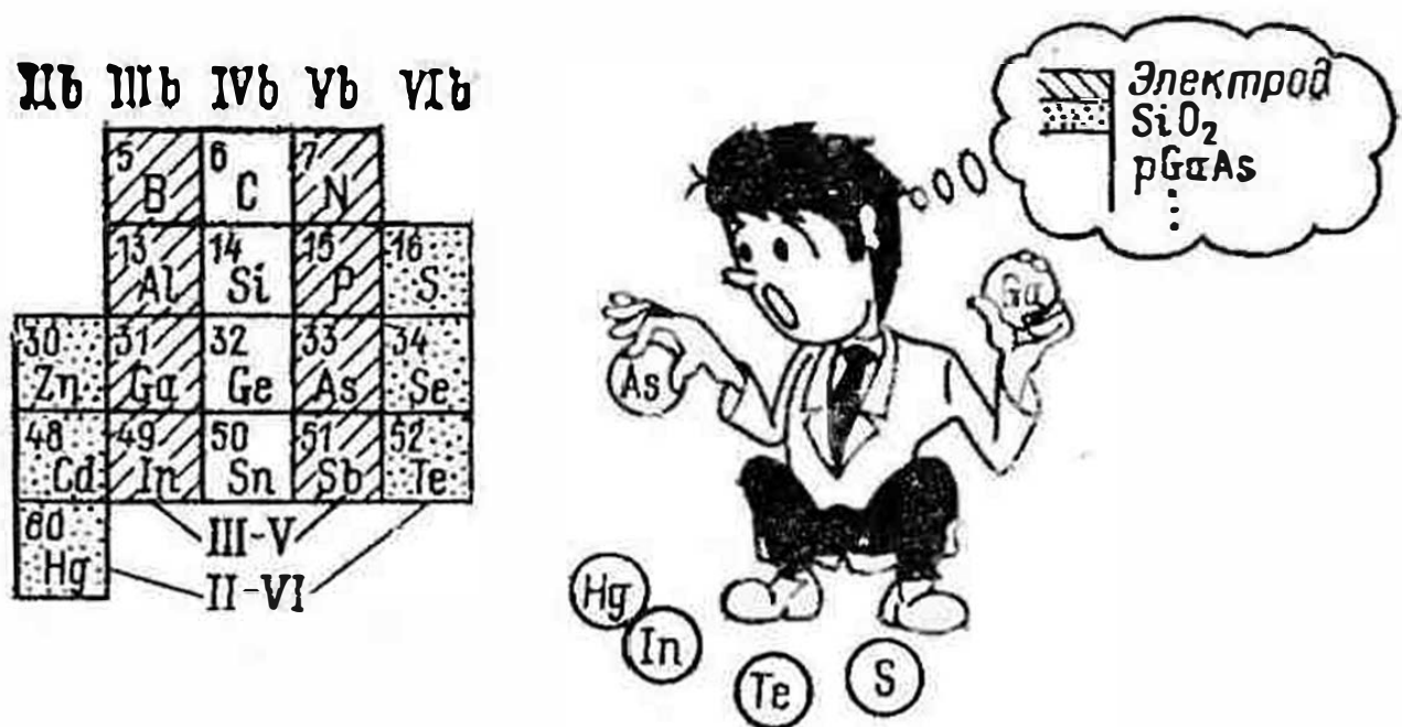
Рис. 35. Химические элементы полупроводниковых соединений
