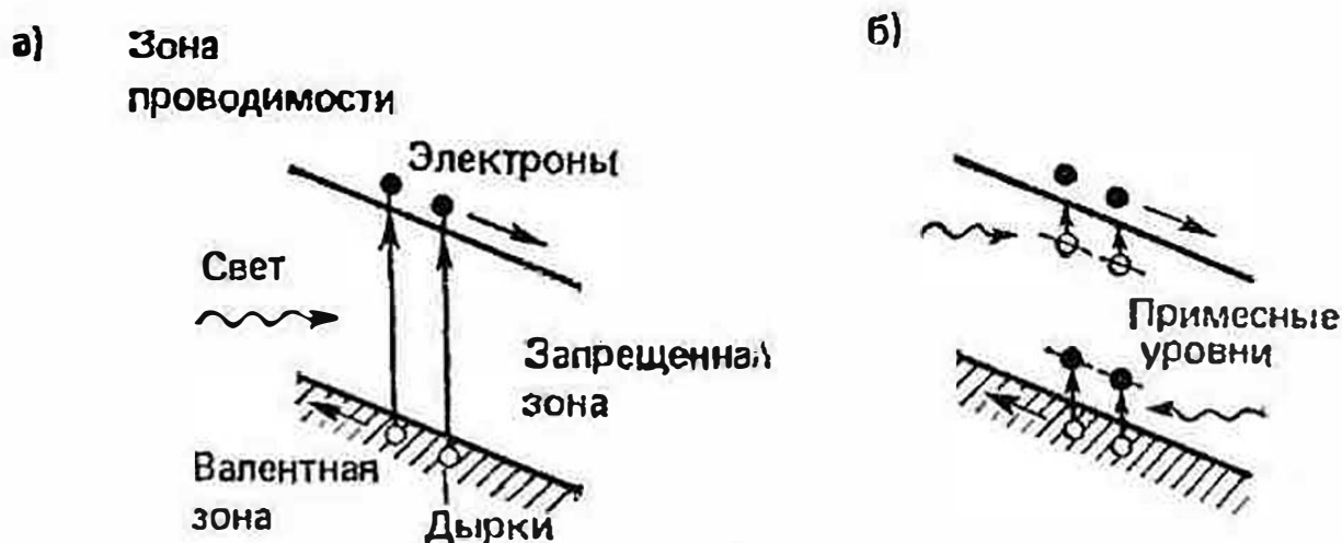
Рис. 28. Механизм фотопроводимости
