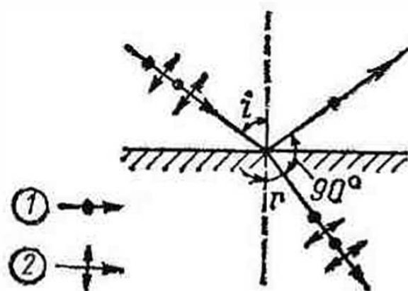
Рис. 10. Поляризация отраженного света
