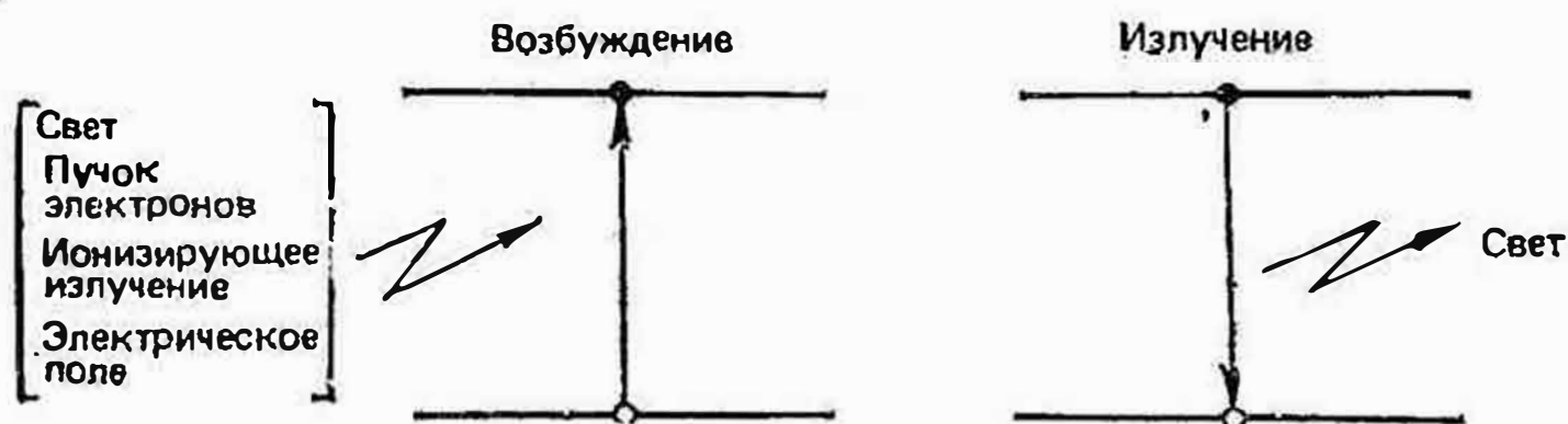
Рис. 3. Схема люминесценции
