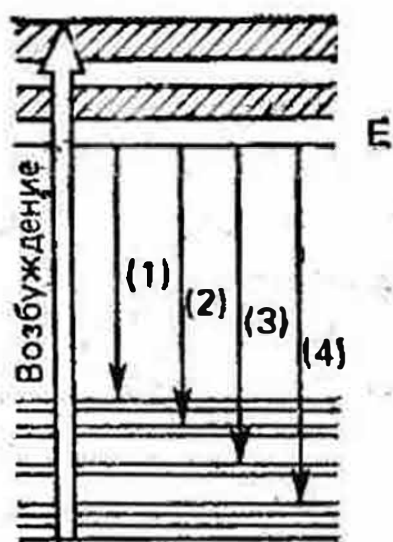
Рис. 65. Диаграмма энергетических уровней \text{YAG}:\text{Nd}^{3+} -лазера
