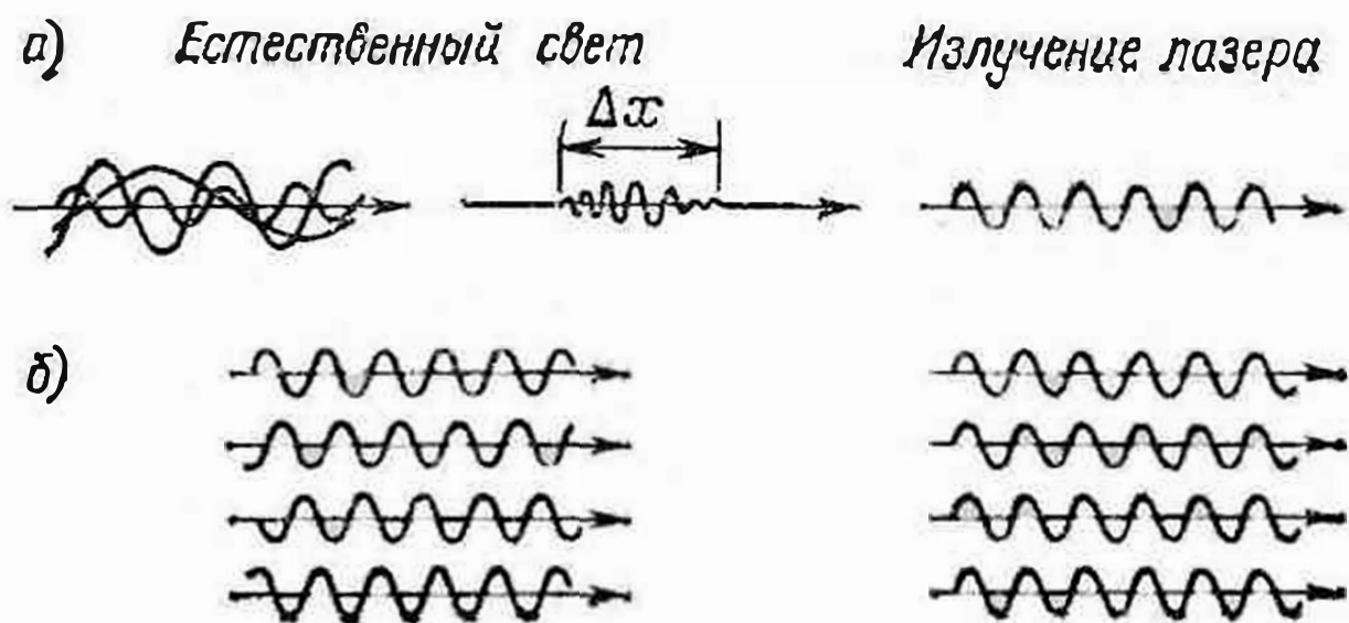
Рис. 12. Временная (а) и пространственная (б) когерентность
