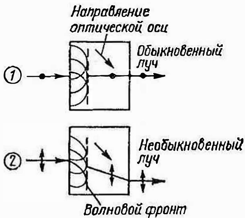
Рис. 11. Двойное лучепреломление
