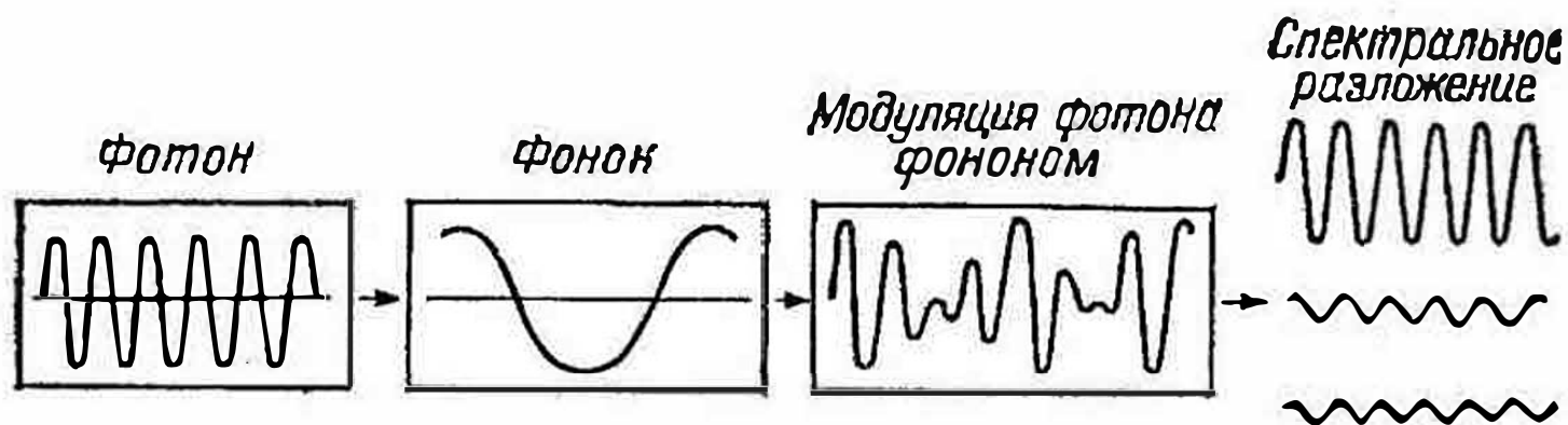
Рис. 22. Эффект Рамана (рассеяние фотона на фононе)
