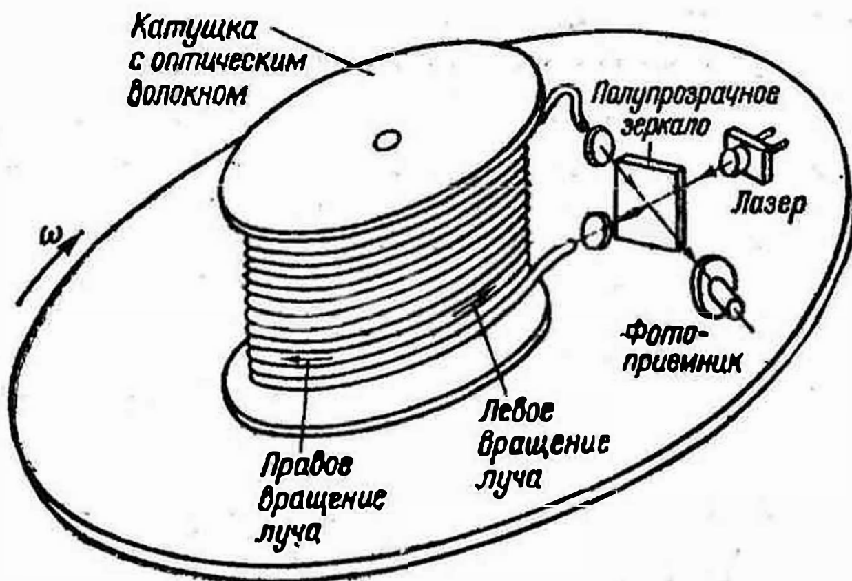
Рис. 139. Волоконно-оптический гироскоп
