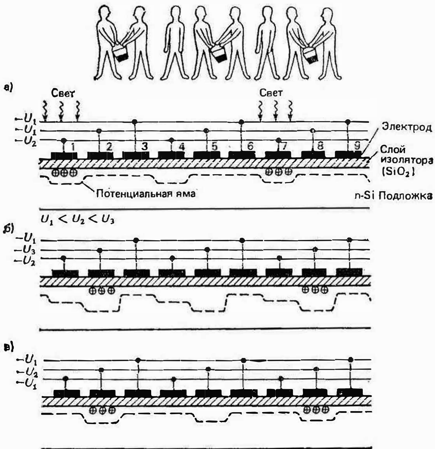
Рис. 95. Принцип работы приборов с зарядовой связью
