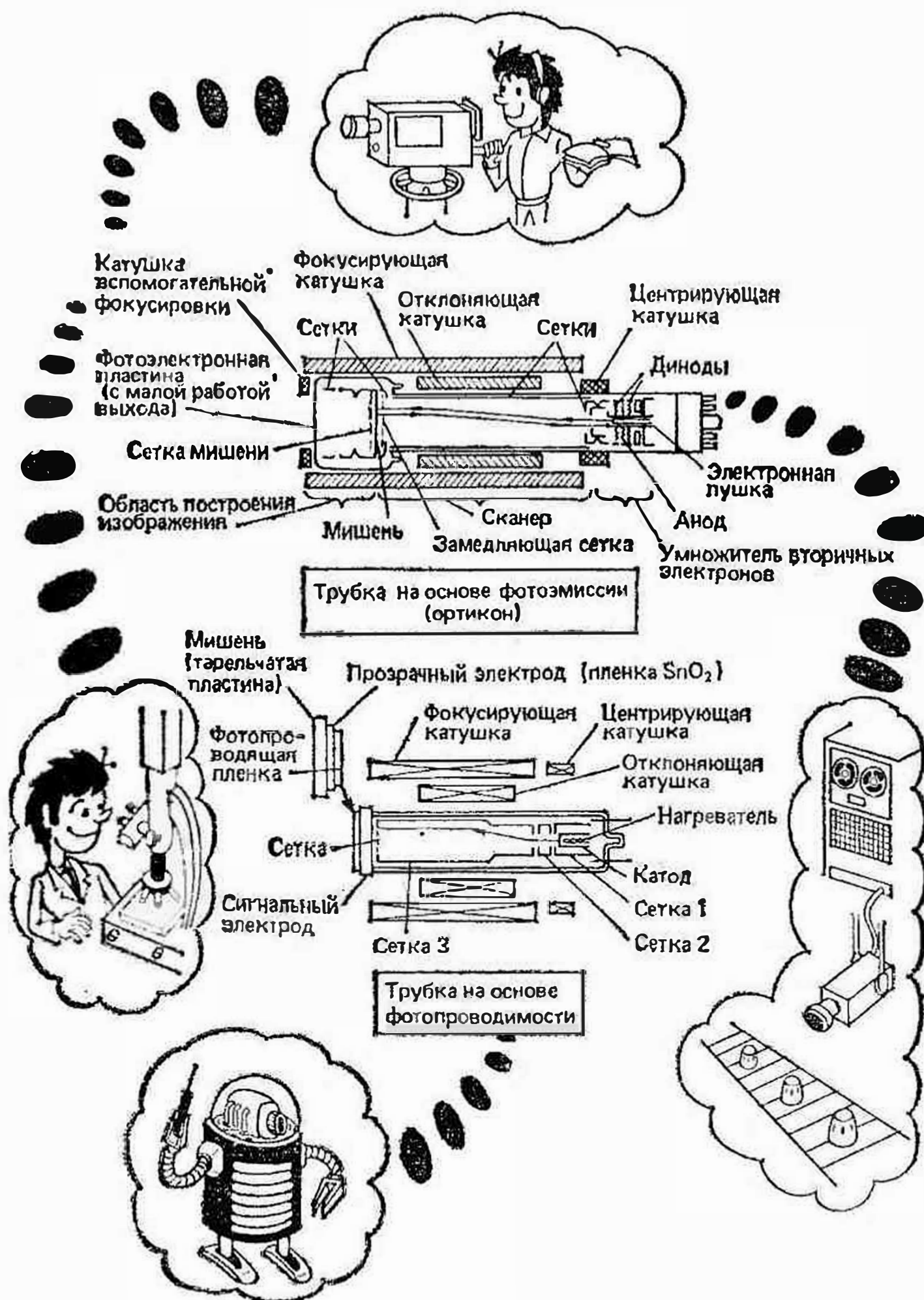
Рис. 94. Передающие телевизионные трубки
