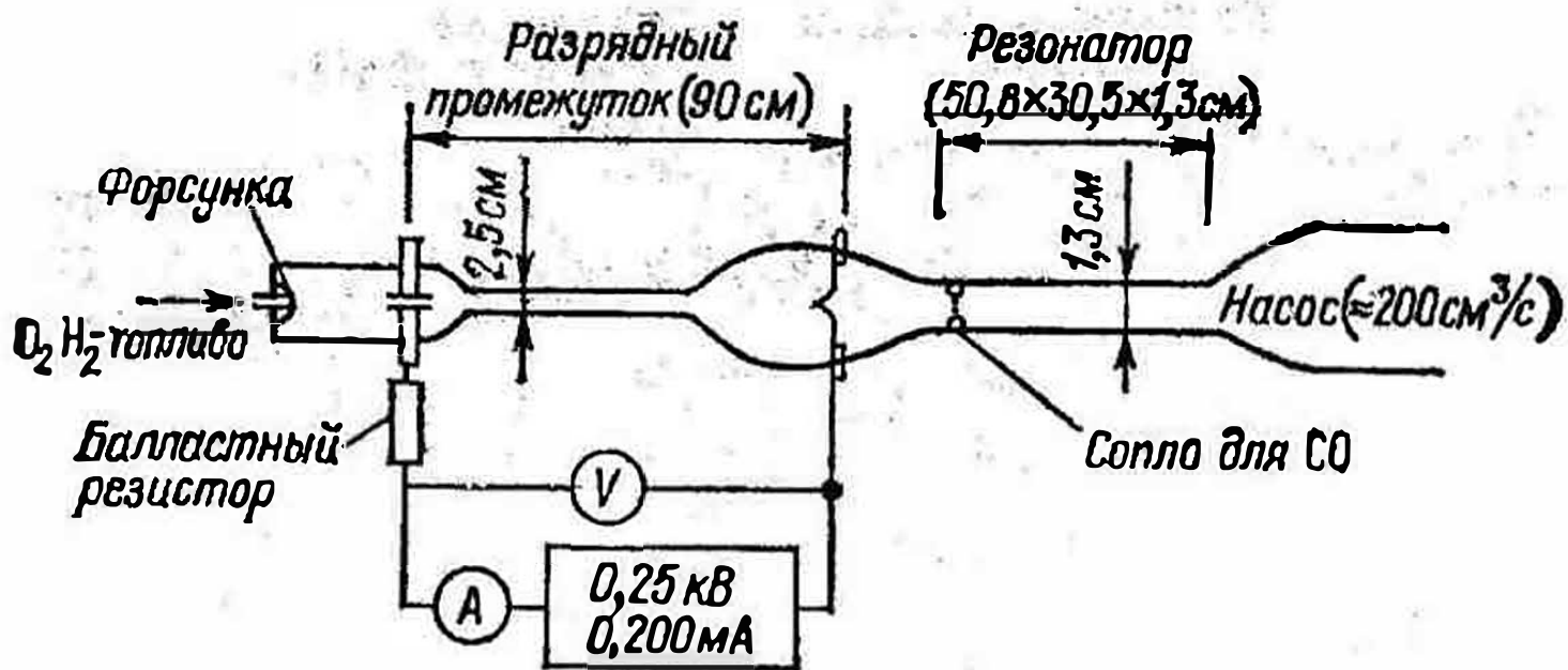
Рис. 61. Лазер на угарном газе
