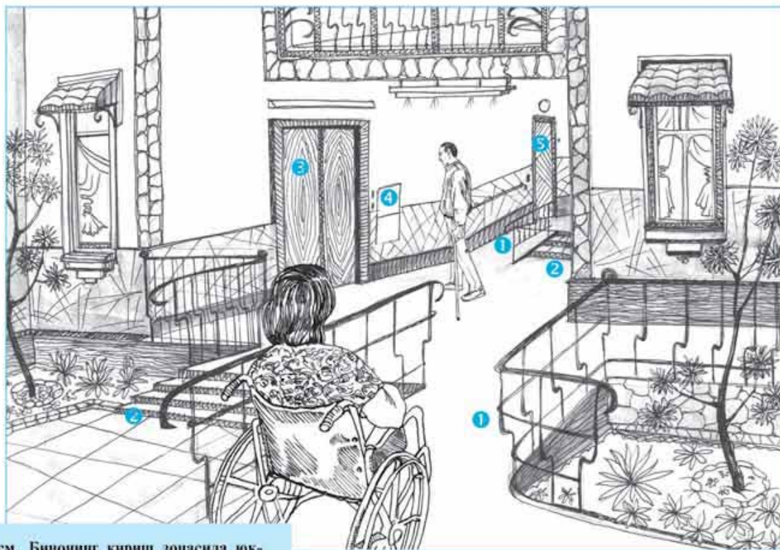
18-расм. Бинонинг кириш зонасида юк-йўловчи лифтининг ташқи киравериши жойлашуви:
