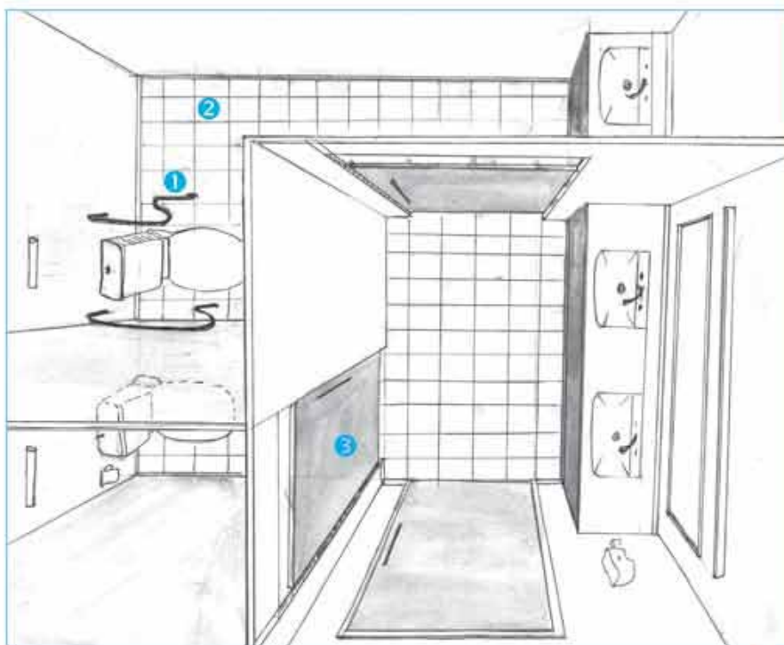
31-расм. Жамоат биноларида ноғиронлиги бор кишилар фойдаланишлари учун мослаштирилган ҳожатхонанинг маҳсуе кабинкалар жойлашуви. Юқоридан кўриниши:
