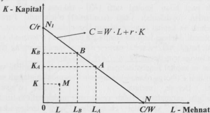
6.9-rasm. Izokosta
