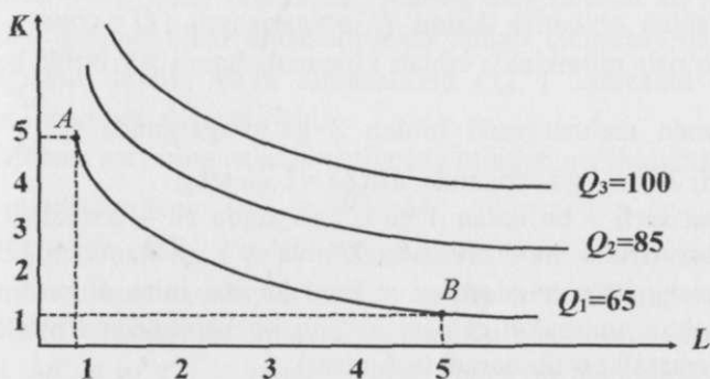
6.5-rasm. Izokvantalar
